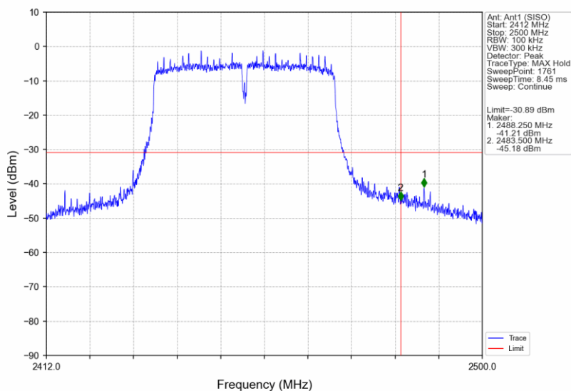
802.11n(HT40)_HCH_2452MHz_Ant1 (SISO)_NTNV
