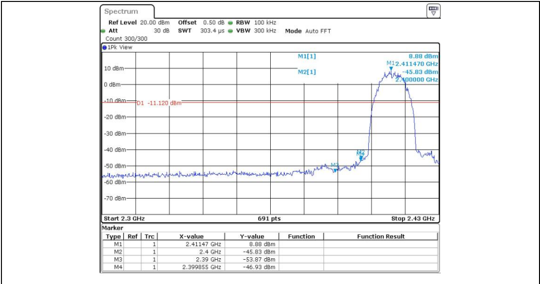
11B_Ant1_Low_2412
