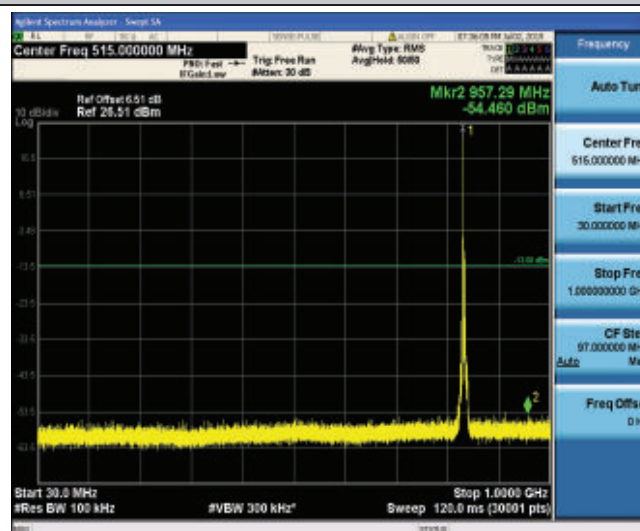
Band5 5MHz QPSK 20525 1RB#0
