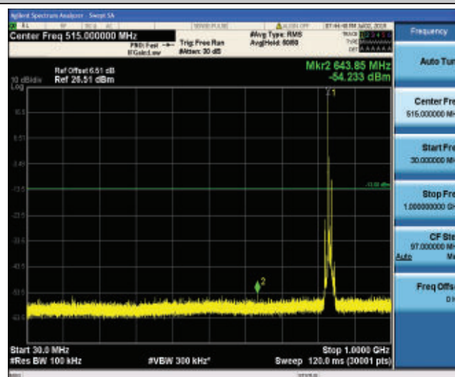
Band5 10MHz QPSK 20525 1RB#0
