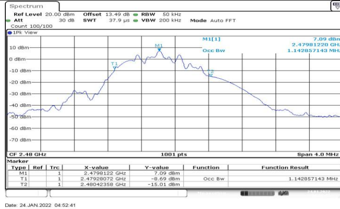
BLE 500K Ant1 2480
