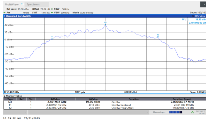
BLE_2M_Ant1_2402
