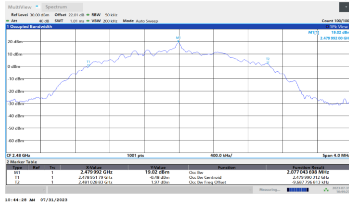
BLE_2M_Ant1_2480
