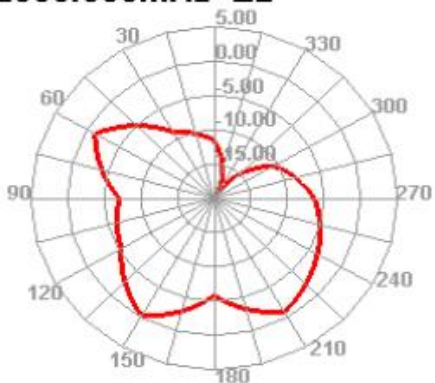
2500.000MHz E2
