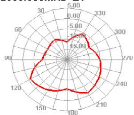
2500.000MHz E1
