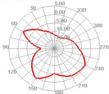
2400.000MHz E2
