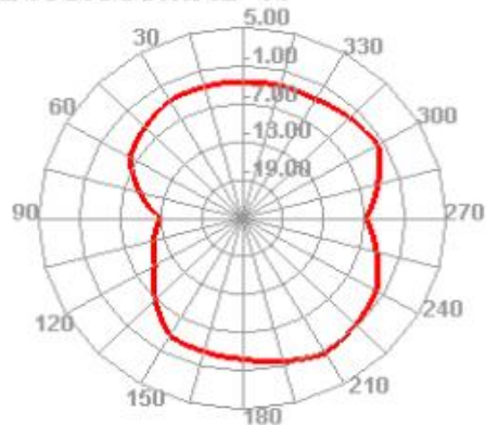
2400.000MHz E2
