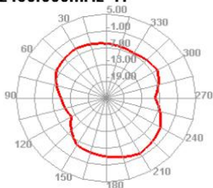
2450.000MHz H
