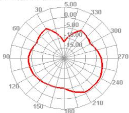
2400.000MHz E1
