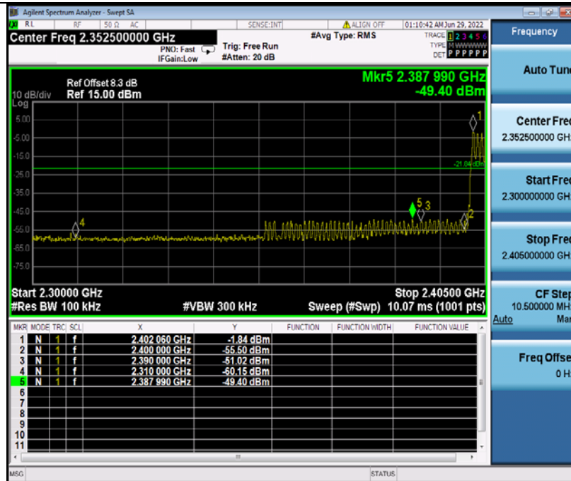
DH5_Ant1_Low_Hop_2402
