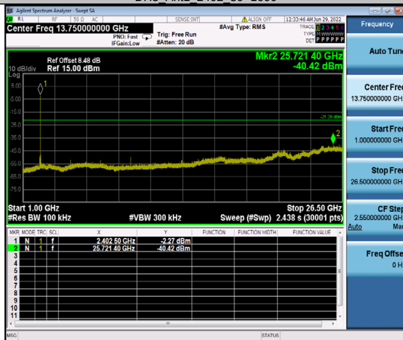
DH5 Ant1_2402_1000~26500
