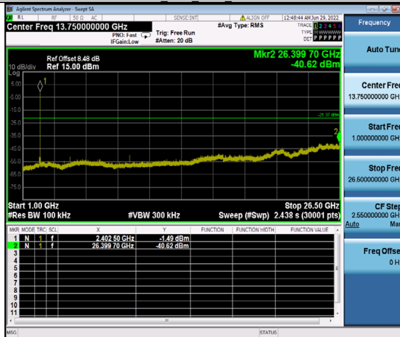
2DH5_Ant1_2402_1000~26500
