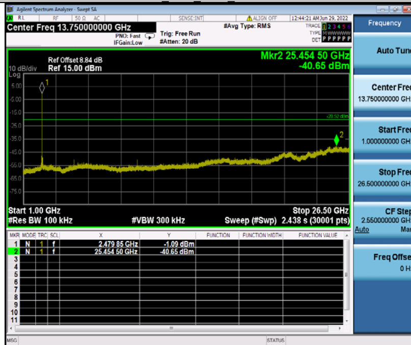
DH5 Ant1_2480_1000~26500
