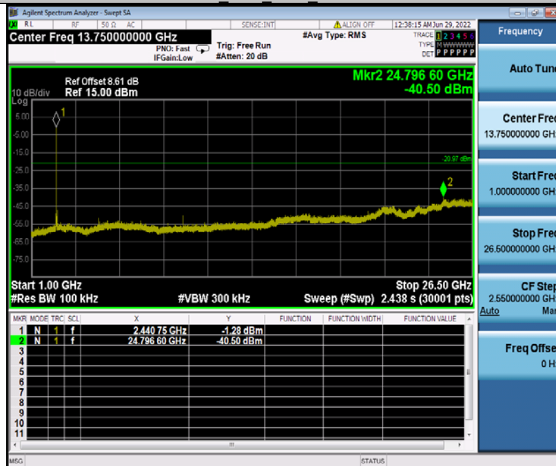
DH5 Ant1_2441_1000~26500
