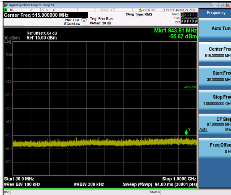
DH5 Ant1_2480_30~1000
