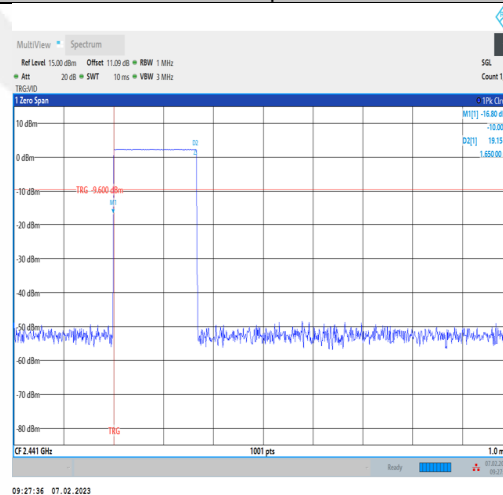
DH3-Ant1-Hop-1.650-160
