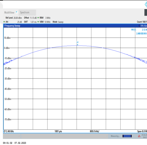
DH5-Ant1-2480
