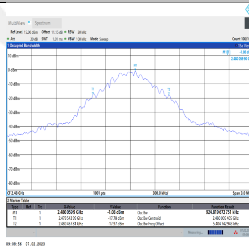
DH5-Ant1-2480
