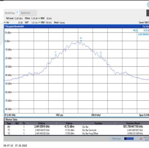
DH5-Ant1-2441
