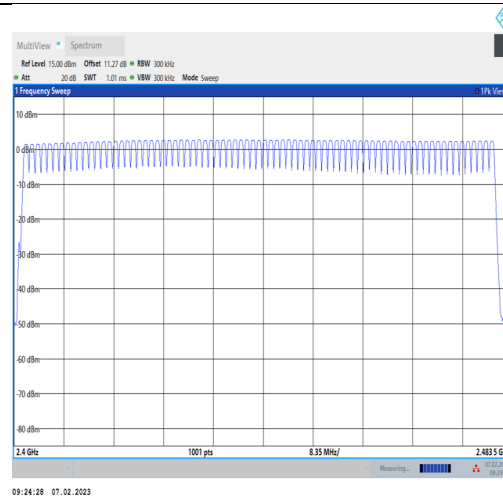
DH5-Ant1-Hop
