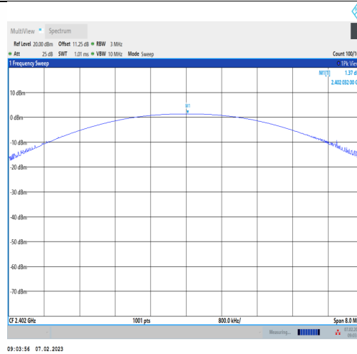
DH5-Ant1-2402
