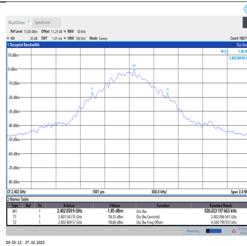
DH5-Ant1-2402
