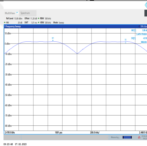
DH5-Ant1-Hop_2480
