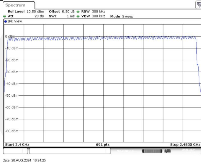
2DH5_Ant1_Hop
