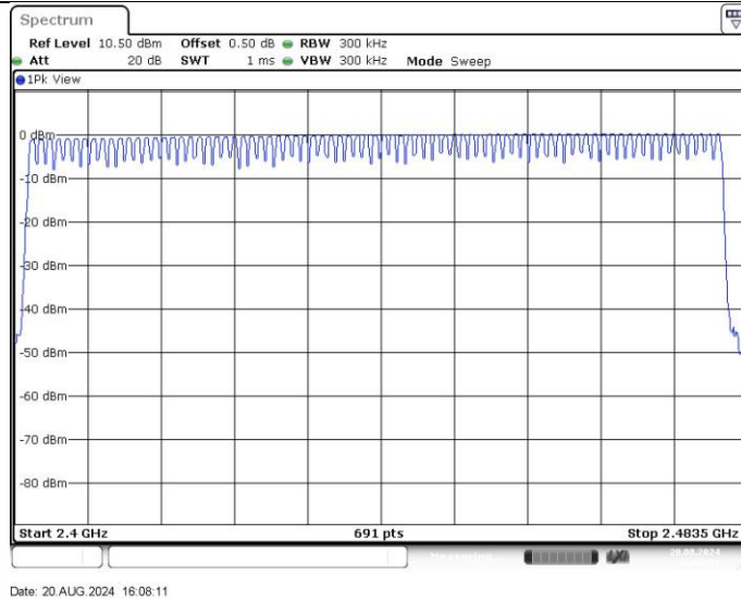
DH5_Ant1_Hop
