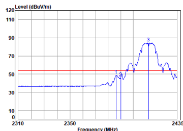
11b_TX_CH_01_Horizontal-Avg
