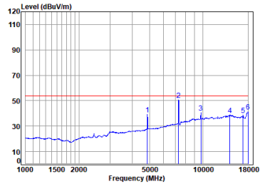
11g_TX_CH_06_Vertical-Avg
