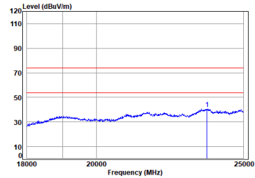
2.4G_SRD_TX_LOW_Vertical
