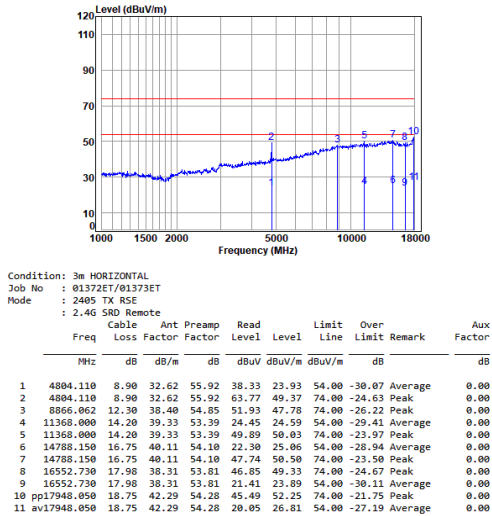
2.4G_SRD_TX_LOW_Horizontal
