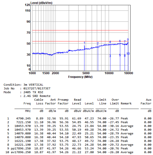
2.4G_SRD_TX_LOW_Vertical
