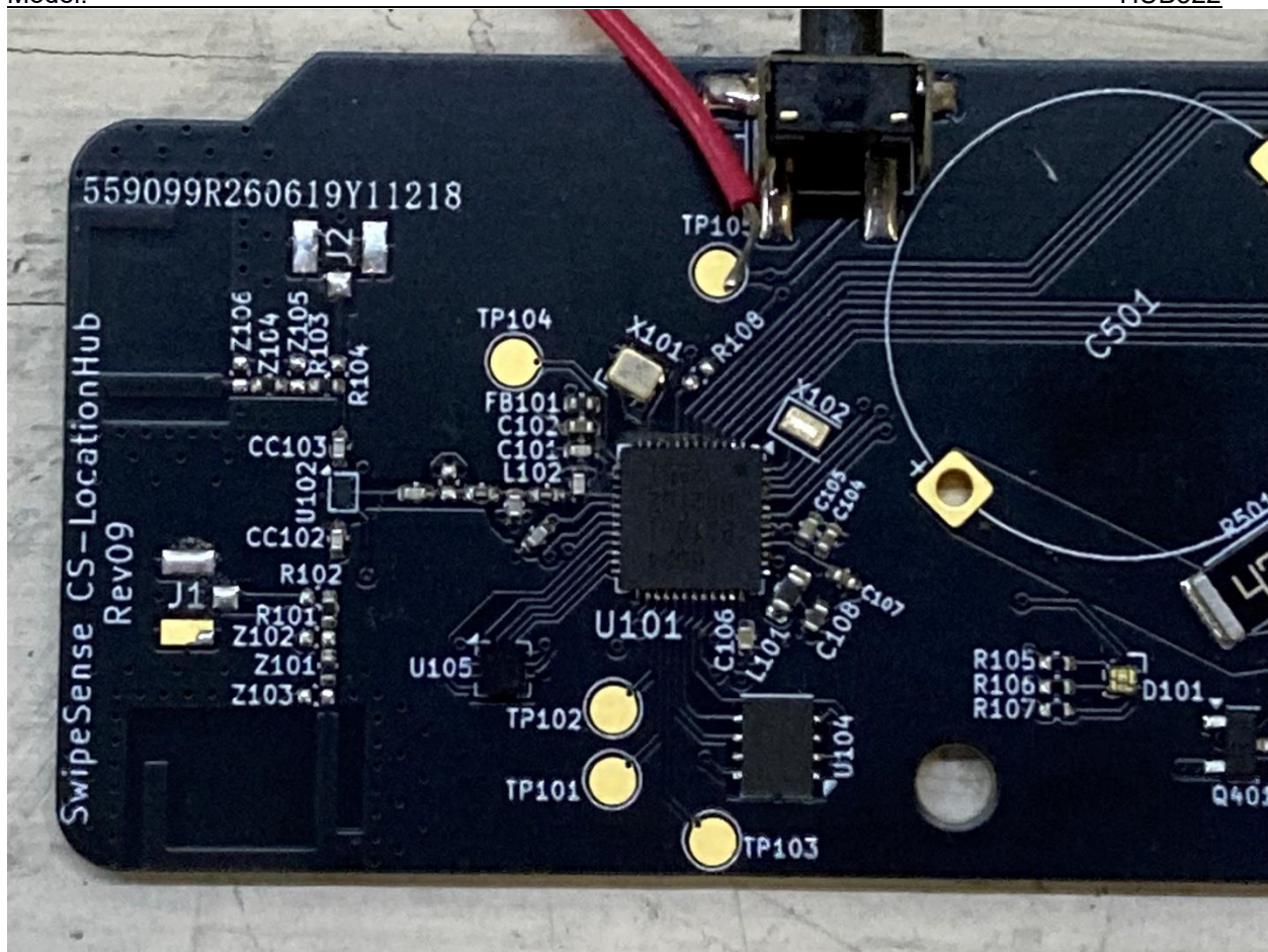
Figure 4. BLE Radio- Close up
