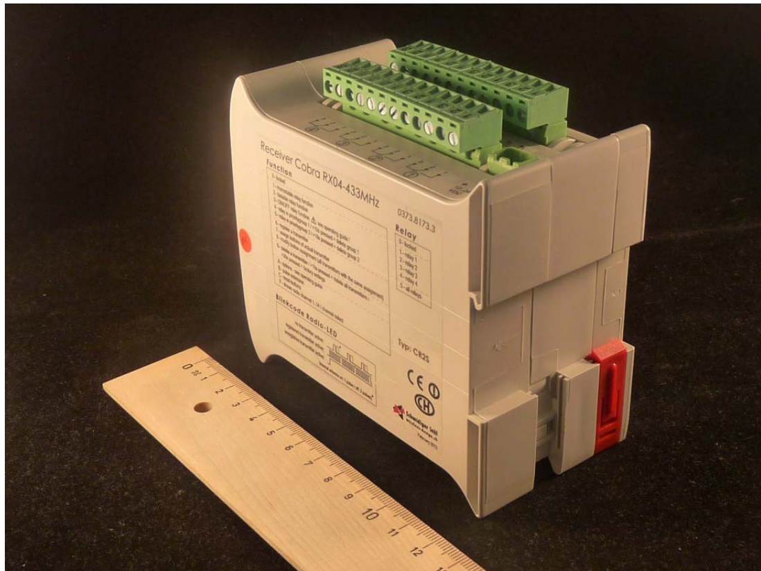
Photo 2: Master Module + Slave Module
