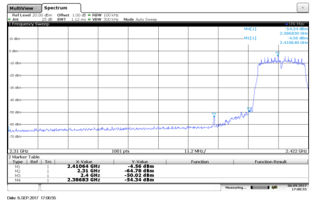
CH01-Bandedge
