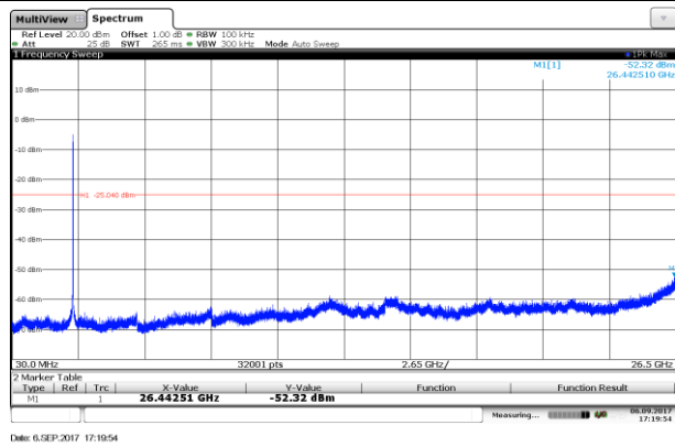
CH09-SE
