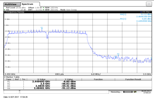
CH09-Bandedge
