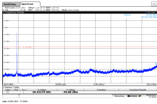
CH03-SE
