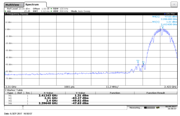
CH01-Bandedge
