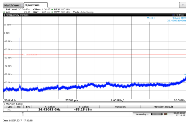
CH06-SE
