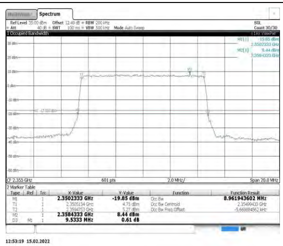
Band40-10MHz-QPSK-39200-50RB#0
