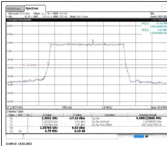
Band40-5MHz-QPSK-38725-25RB#0
