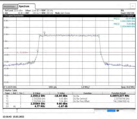
Band40-5MHz-QPSK-39225-25RB#0
