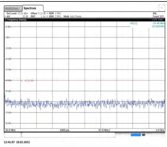
Band40-5MHz-QPSK-38750-1RB#0- Range1:30~1000MHz
