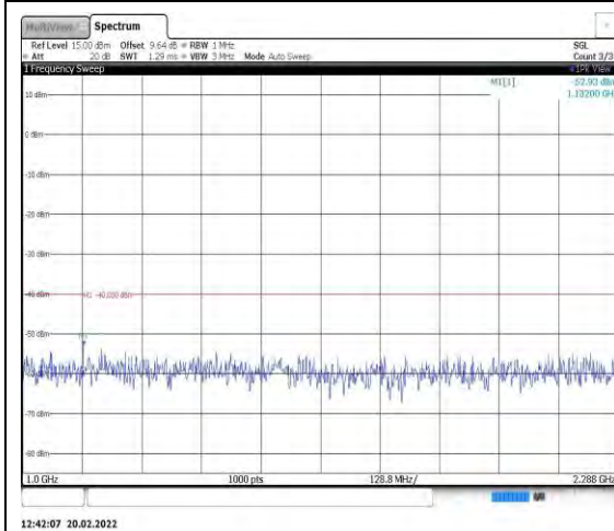
Band40-5MHz-QPSK-38750-1RB#0- Range2:1000~2288MHz
