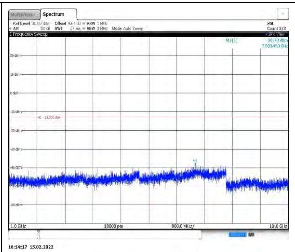
Band26-1.4MHz-QPSK-26697-1RB#0- Range2:1000~10000MHz
