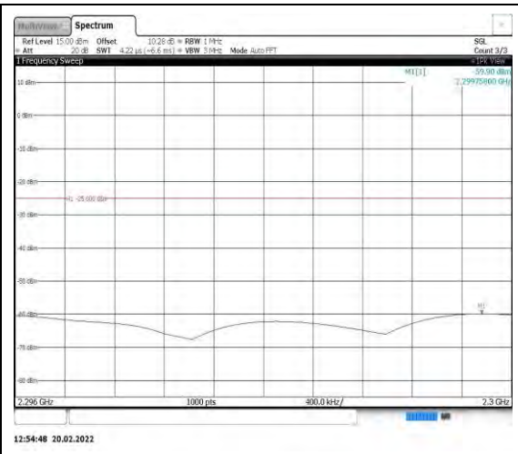
Band40-5MHz-QPSK-39175-1RB#0- Range5:2296~2300MHz
