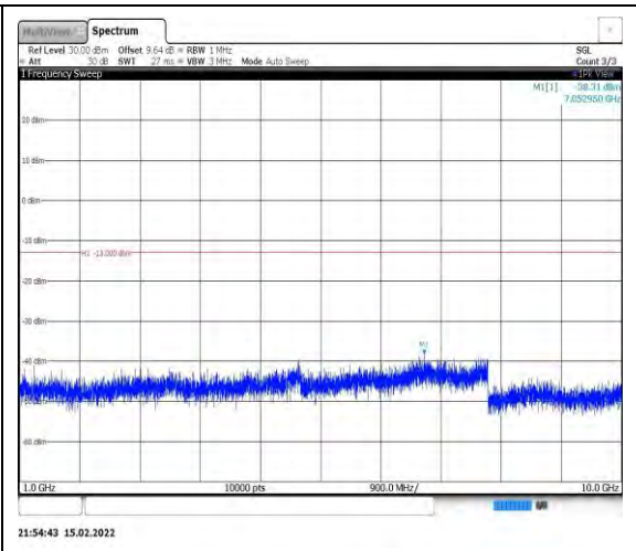
Band26-5MHz-QPSK-26715-1RB#0- Range2:1000~10000MHz
