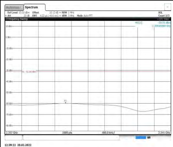
Band40-5MHz-QPSK-38725-1RB#0- Range10:2337~2341MHz
