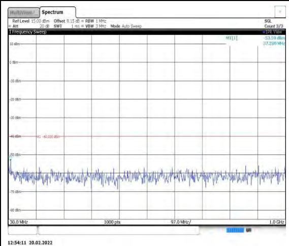
Band40-5MHz-QPSK-39175-1RB#0- Range1:30~1000MHz
