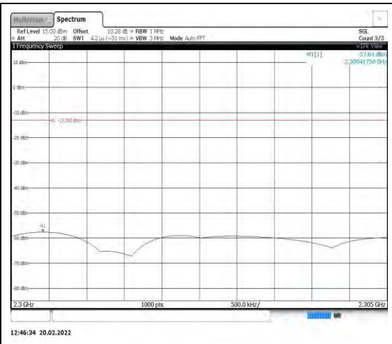
Band40-5MHz-QPSK-38775-1RB#0- Range6:2300~2305MHz
