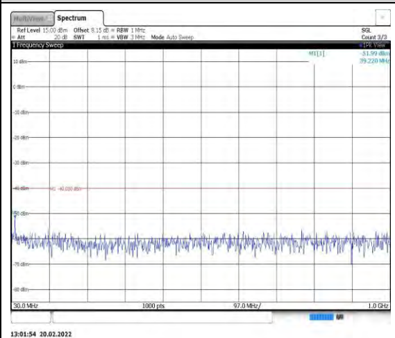
Band40-5MHz-QPSK-39225-1RB#0- Range1:30~1000MHz
