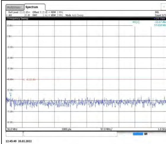
Band40-5MHz-QPSK-38775-1RB#0- Range1:30~1000MHz
