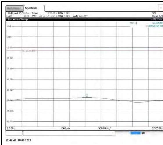
Band40-5MHz-QPSK-38750-1RB#0- Range6:2300~2305MHz
