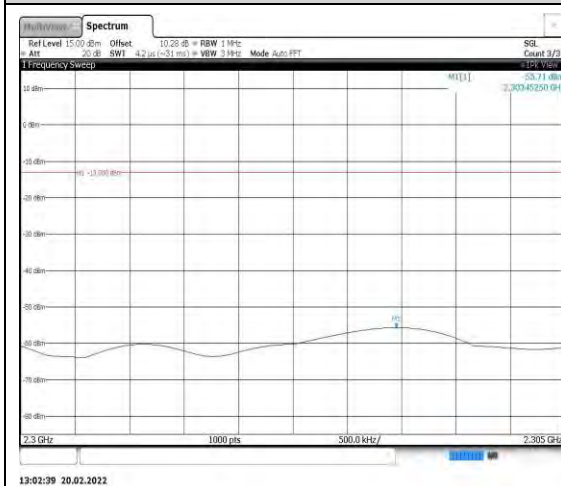
Band40-5MHz-QPSK-39225-1RB#0- Range6:2300~2305MHz
