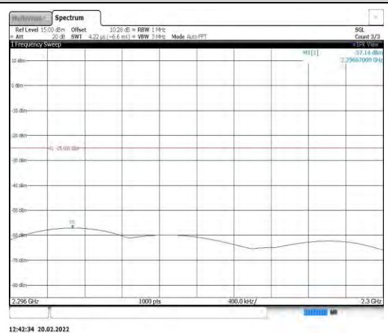
Band40-5MHz-QPSK-38750-1RB#0- Range5:2296~2300MHz
