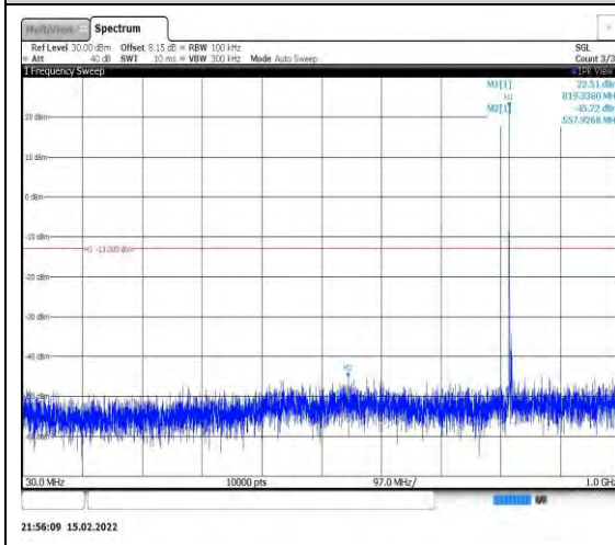
Band26-5MHz-QPSK-26765-1RB#0- Range1:30~1000MHz
