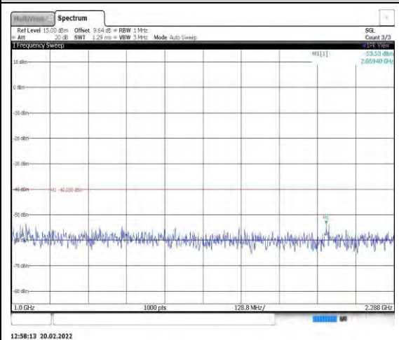
Band40-5MHz-QPSK-39200-1RB#0- Range2:1000~2288MHz
