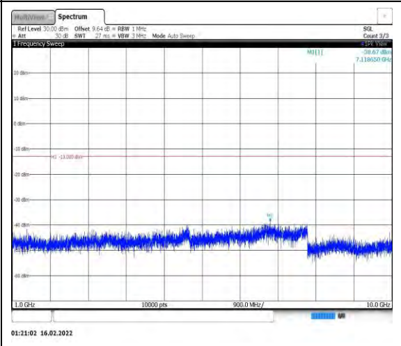
Band26-3MHz-QPSK-27025-1RB#0- Range2:1000~10000MHz
