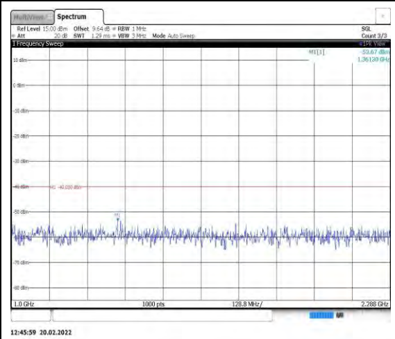
Band40-5MHz-QPSK-38775-1RB#0- Range2:1000~2288MHz
