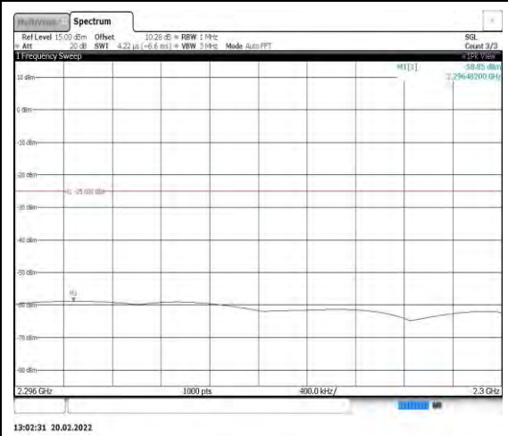
Band40-5MHz-QPSK-39225-1RB#0- Range5:2296~2300MHz
