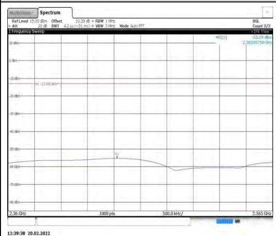
Band40-5MHz-QPSK-38725-1RB#0- Range12:2360~2365MHz
