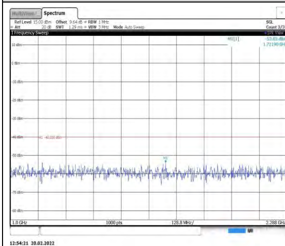
Band40-5MHz-QPSK-39175-1RB#0- Range2:1000~2288MHz
