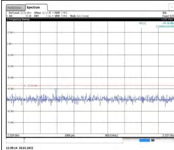
Band40-5MHz-QPSK-38725-1RB#0- Range9:2328~2337MHz
