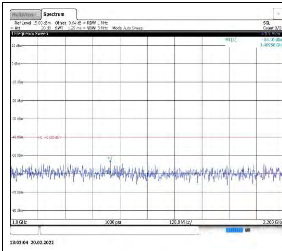
Band40-5MHz-QPSK-39225-1RB#0- Range2:1000~2288MHz
