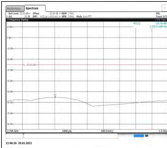
Band40-5MHz-QPSK-38775-1RB#0- Range5:2296~2300MHz
