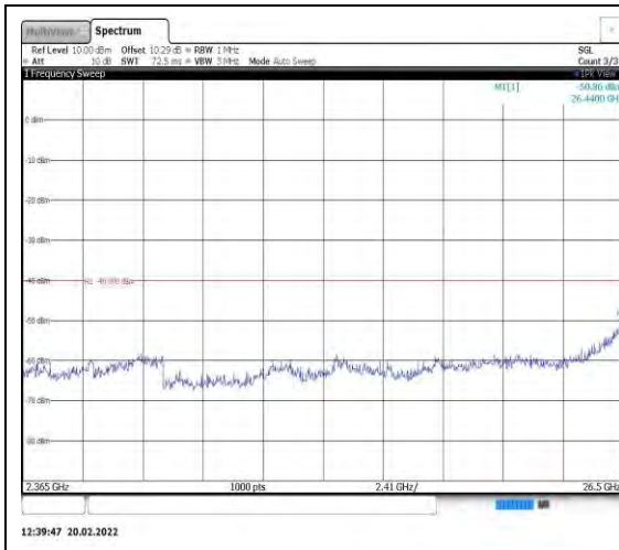
Band40-5MHz-QPSK-38725-1RB#0- Range13:2365~26500MHz
