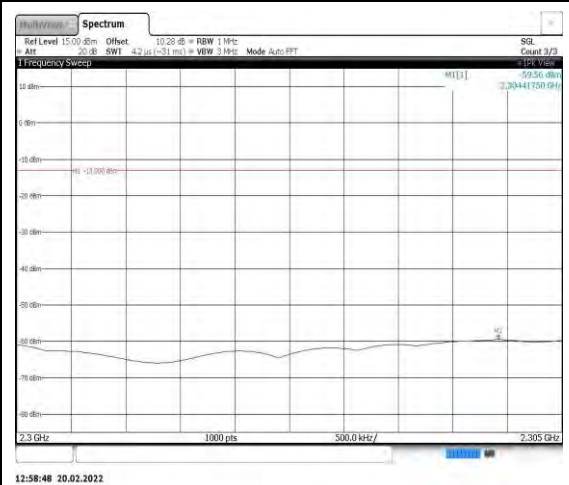
Band40-5MHz-QPSK-39200-1RB#0- Range6:2300~2305MHz
