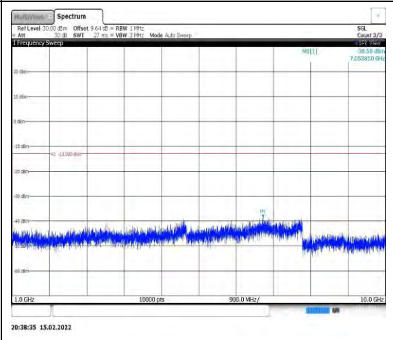
Band26-3MHz-QPSK-26775-1RB#0- Range2:1000~10000MHz
