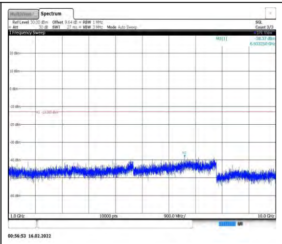
Band26-1.4MHz-QPSK-26797-1RB#0- Range2:1000~10000MHz
