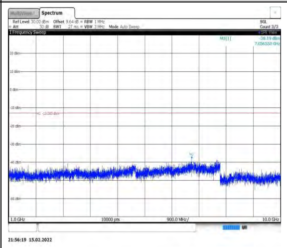
Band26-5MHz-QPSK-26765-1RB#0- Range2:1000~10000MHz
