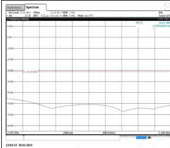
Band40-5MHz-QPSK-39225-1RB#0- Range4:2292~2296MHz
