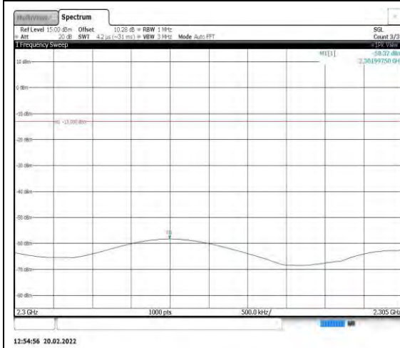
Band40-5MHz-QPSK-39175-1RB#0- Range6:2300~2305MHz
