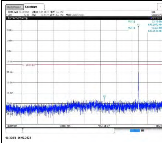
Band26-3MHz-QPSK-27025-1RB#0- Range1:30~1000MHz
