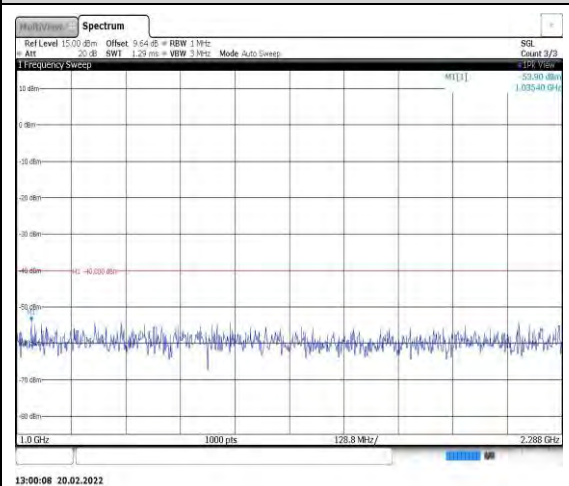
Band40-5MHz-16QAM-39200-1RB#0- Range2:1000~2288MHz
