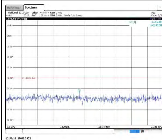
Band40-5MHz-16QAM-39175-1RB#0- Range2:1000~2288MHz
