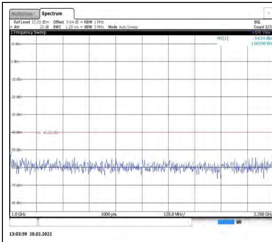
Band40-5MHz-16QAM-39225-1RB#0- Range2:1000~2288MHz
