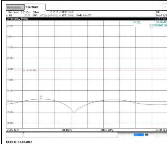
Band40-5MHz-QPSK-39225-1RB#0- Range10:2337~2341MHz
