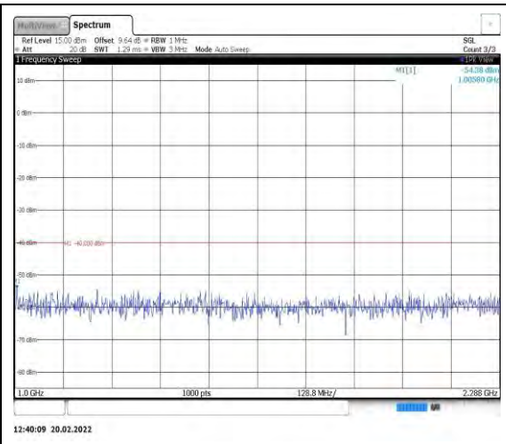
Band40-5MHz-16QAM-38725-1RB#0- Range2:1000~2288MHz
