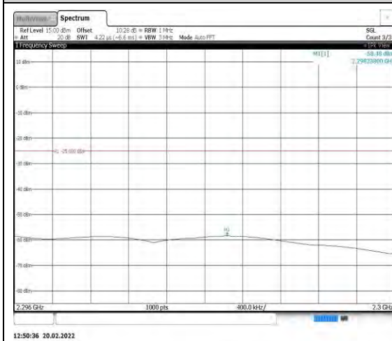
Band40-10MHz-QPSK-38750-1RB#0- Range5:2296~2300MHz
