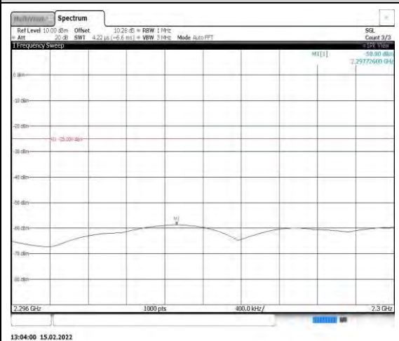
Band40-10MHz-QPSK-39200-1RB#0- Range5:2296~2300MHz
