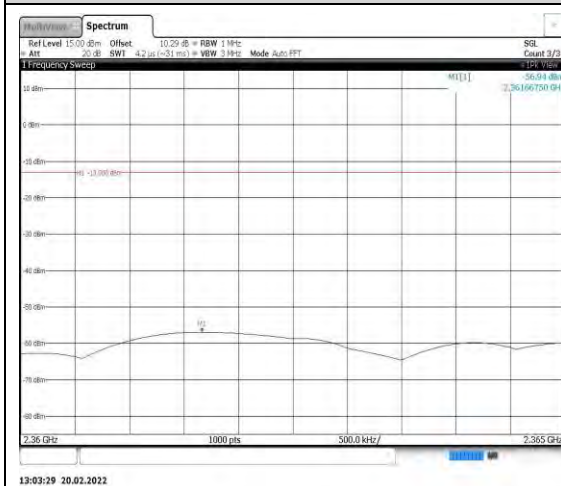
Band40-5MHz-QPSK-39225-1RB#0- Range12:2360~2365MHz
