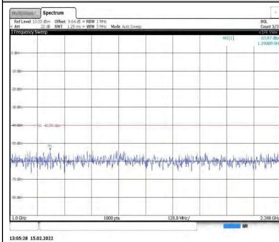
Band40-10MHz-16QAM-39200-1RB#0- Range2:1000~2288MHz
