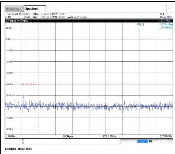
Band40-10MHz-QPSK-38750-1RB#0- Range2:1000~2288MHz
