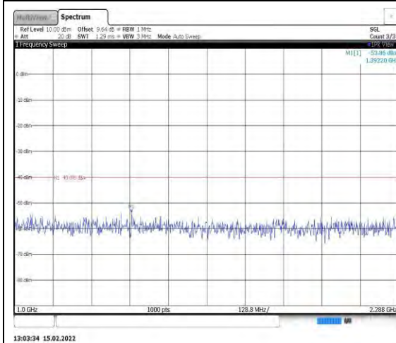
Band40-10MHz-QPSK-39200-1RB#0- Range2:1000~2288MHz
