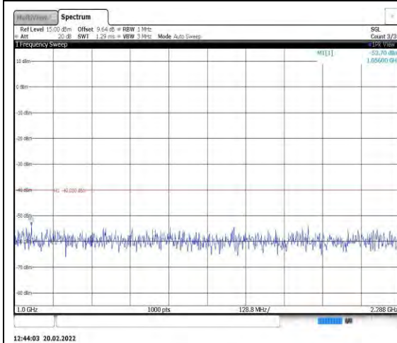
Band40-5MHz-16QAM-38750-1RB#0- Range2:1000~2288MHz
