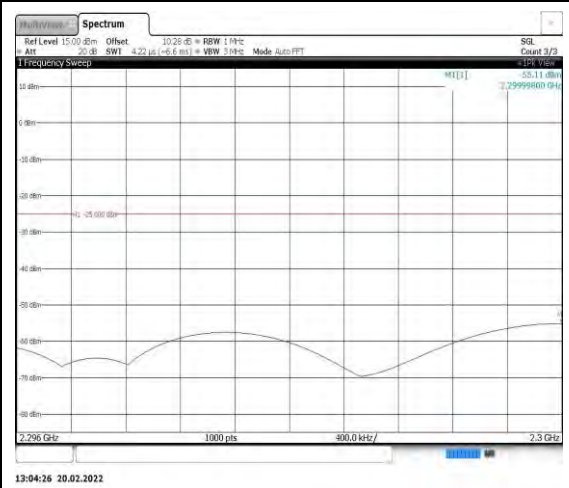
Band40-5MHz-16QAM-39225-1RB#0- Range5:2296~2300MHz
