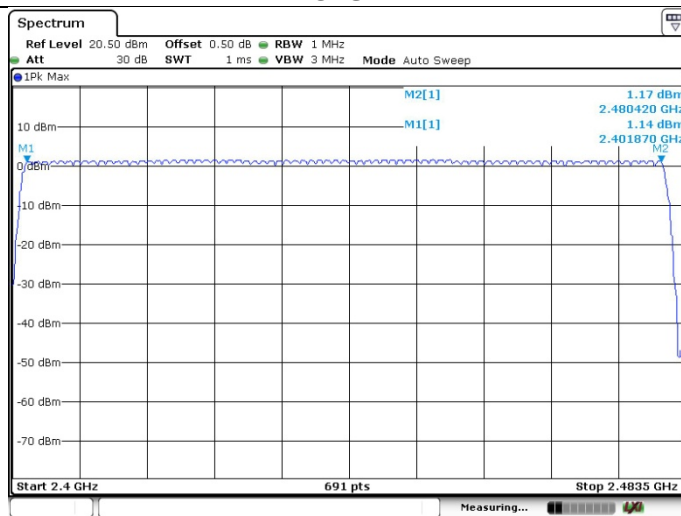
\pi/4 DQPSK
