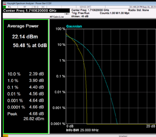
QPSK-20350
