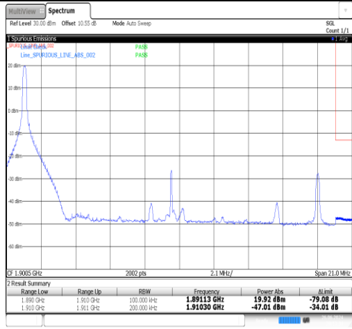
Band2-20MHz-16QAM-19100-1RB#99-PASS
