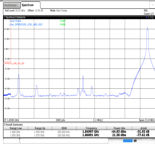
Band2-20MHz-QPSK-19100-100RB#0-PASS
