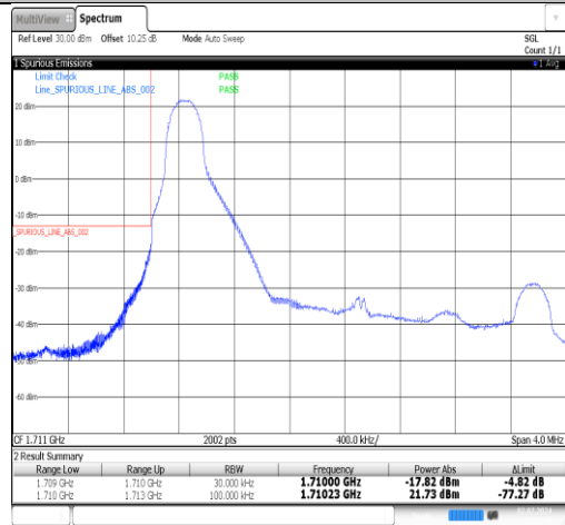
Band4-3MHz-QPSK-19965-1RB#14-PASS
