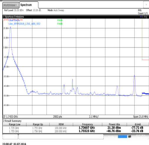
Band4-20MHz-QPSK-20300-1RB#99-PASS
