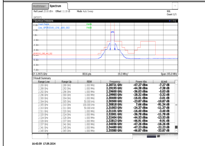
40(2305-2315)-5MHz-QPSK-38775-1RB#0-PASS
