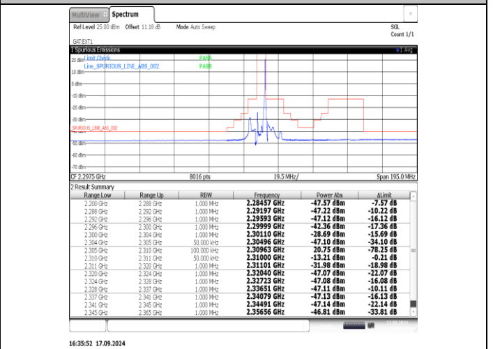
40(2305-2315)-5MHz-QPSK-38775-25RB#0-PASS
