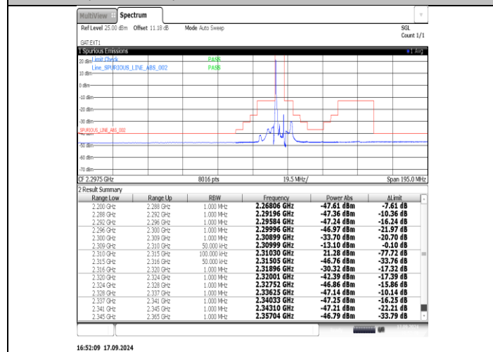
40(2305-2315)-5MHz-QPSK-38775-1RB#24-PASS
