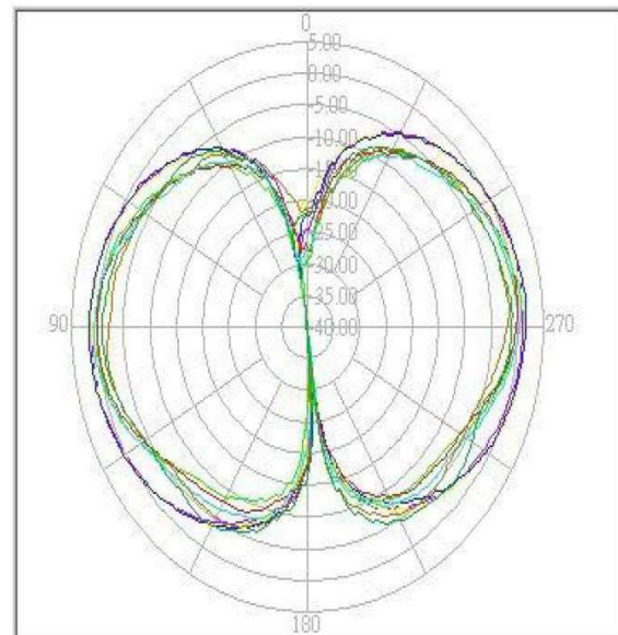
E-Plane
