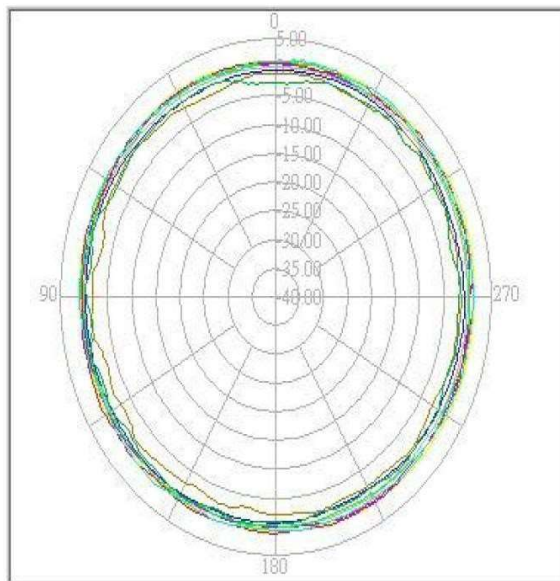
H-Plane
