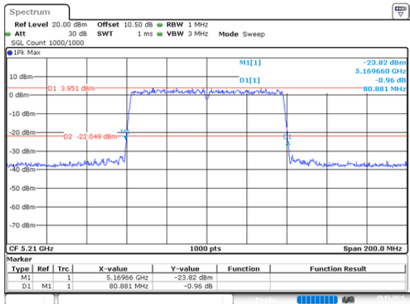
ac80_5210MHz_Chain 0 80.881MHz
