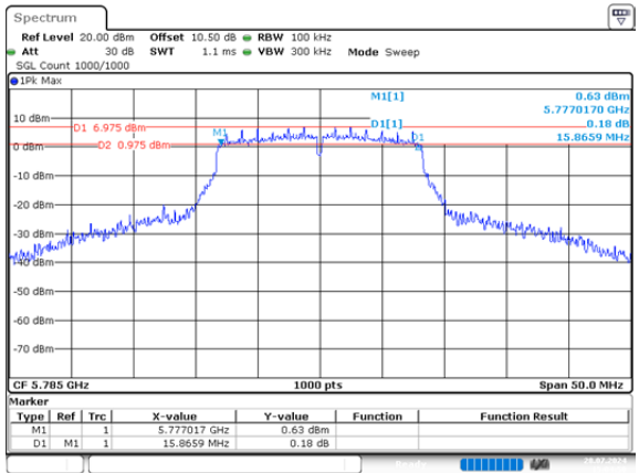
a_5785MHz_Chain 1 15.866MHz
