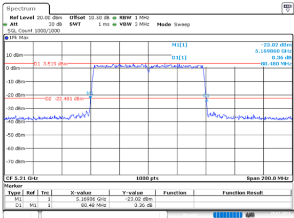
ac80_5210MHz_Chain 1 80.480MHz
