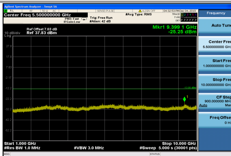
EGPRS850-251-1000~10000
