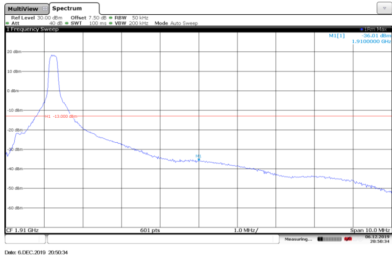
Band2-5MHz-QPSK-19175-1RB#
