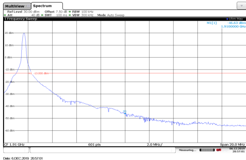
Band2-10MHz-QPSK-19150-1RB#
