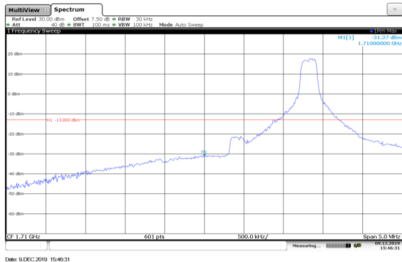
Band4-3MHz-QPSK-19965-1RB#
