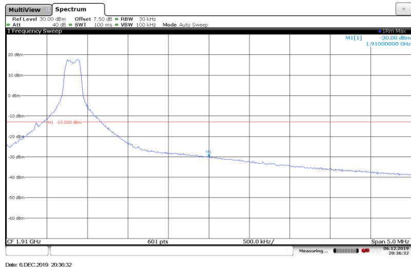
Band2-3MHz-QPSK-19185-1RB#
