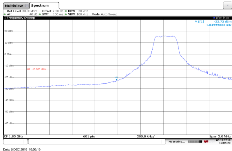
Band2-3MHz-QPSK-18615-1RB#
