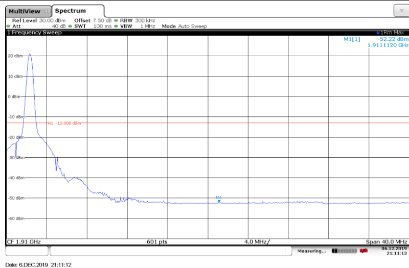
Band2-20MHz-16QAM-19100-1RB#
