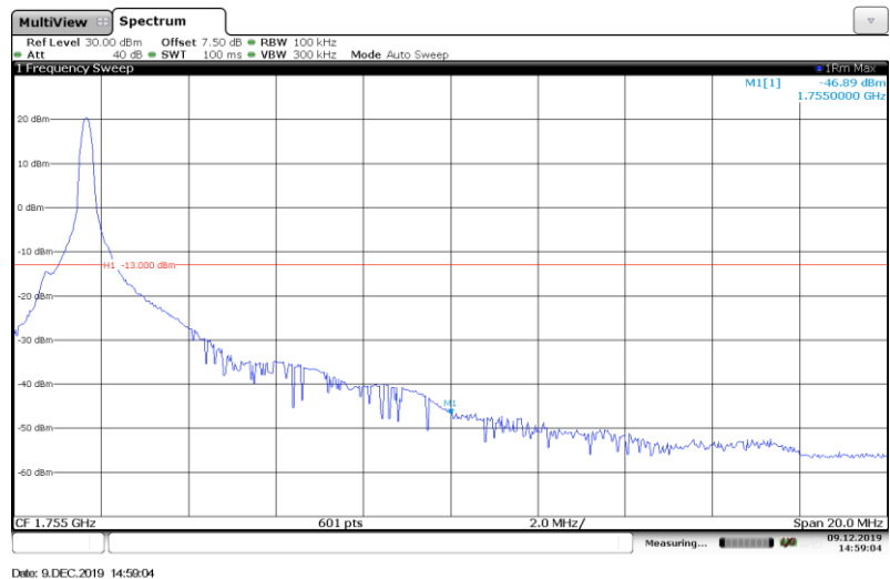
Band4-10MHz-QPSK-20350-1RB#
