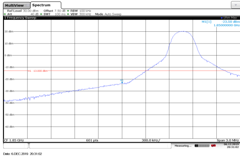
Band2-10MHz-QPSK-18650-1RB#
