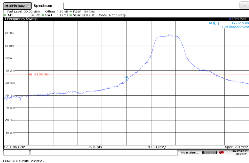
Band2-5MHz-QPSK-18625-1RB#
