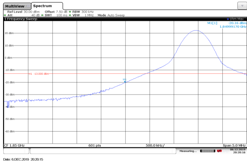
Band2-20MHz-16QAM-18700-1RB#
