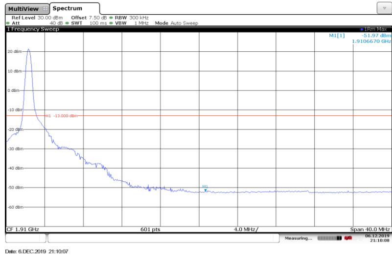
Band2-20MHz-QPSK-19100-1RB#
