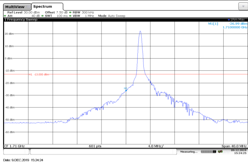
Band4-20MHz-QPSK-20050-1RB#
