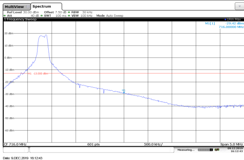
Band12-3MHz-QPSK-23165-1RB#
