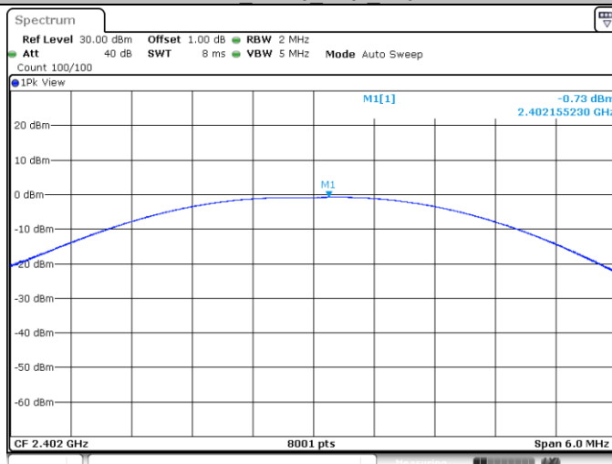
BLE BT4.0 Ant1_2402
