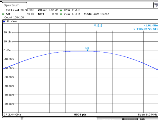
BLE BT4.0 Ant1_2440
