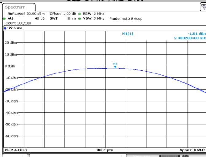
BLE BT4.0 Ant1_2480
