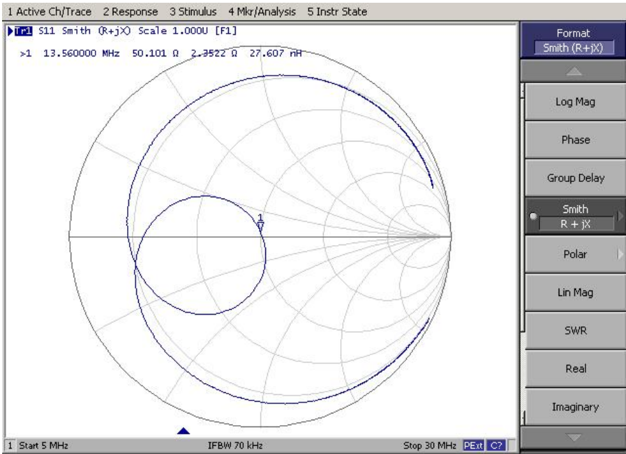
史密斯图
