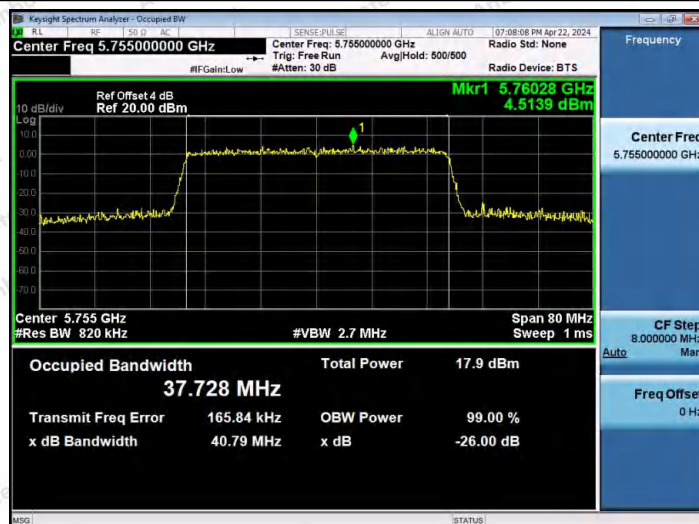
11AX40MIMO-Ant1-5755
