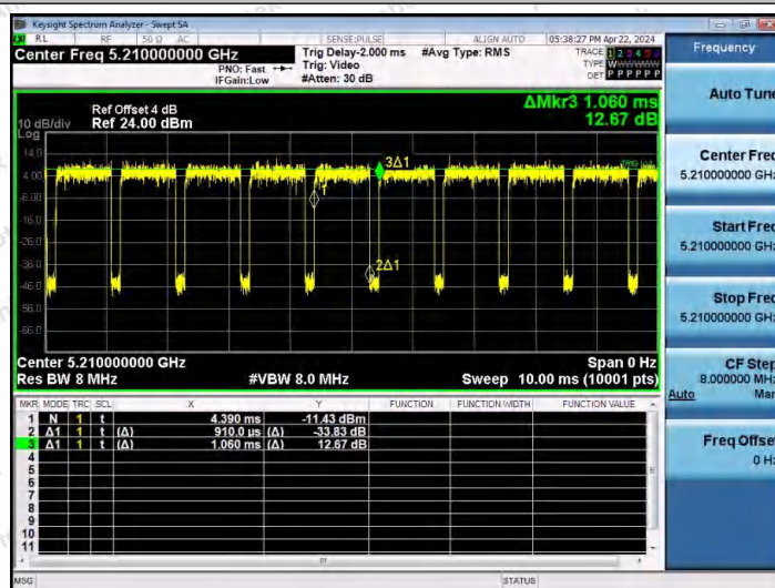
NTNV-11AC80MIMO-Ant1-5210
