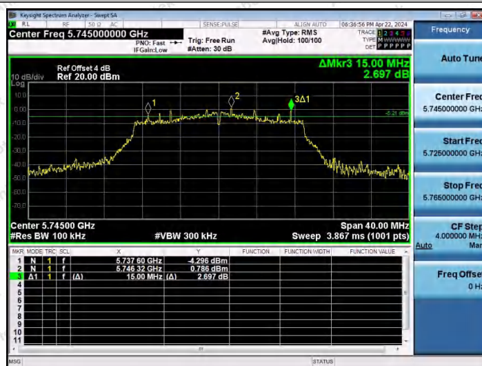
11A20MIMO-Ant1-5745-PASS
