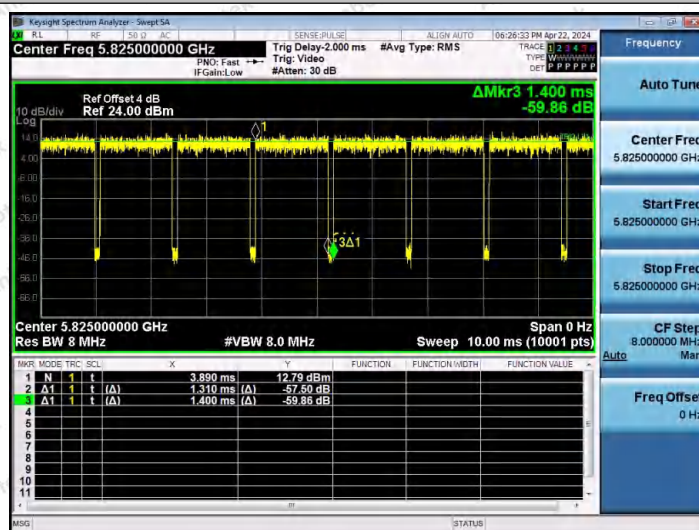
NTNV-11N20MIMO-Ant1-5825
