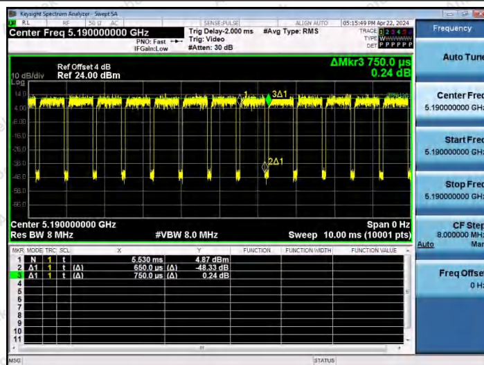
NTNV-11N40MIMO-Ant1-5190
