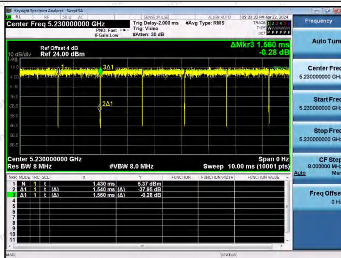
NTNV-11AC40MIMO-Ant1-5230
