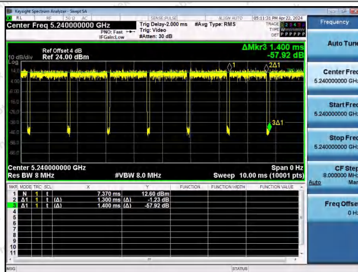
NTNV-11N20MIMO-Ant1-5240
