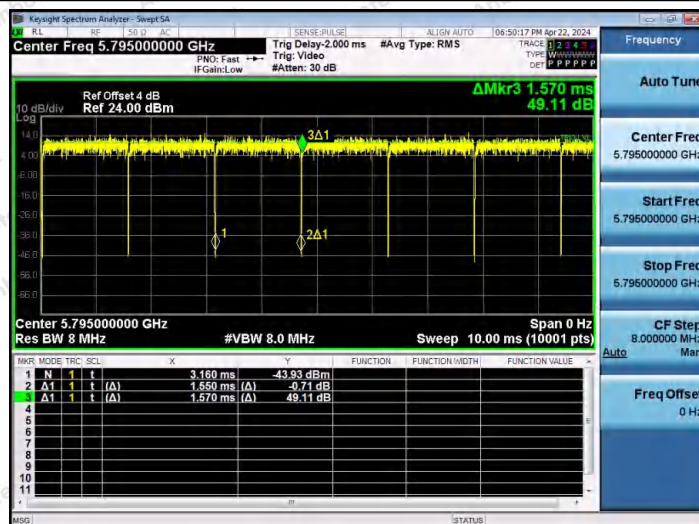
NTNV-11AC40MIMO-Ant1-5795
