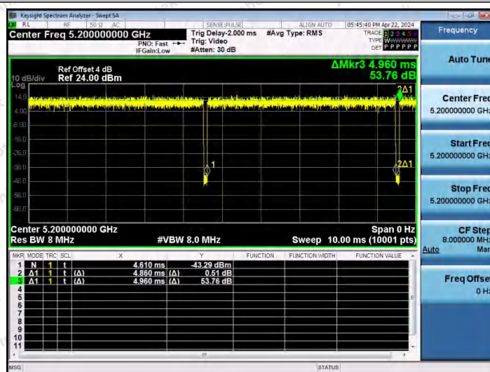
NTNV-11AX20MIMO-Ant1-5200
