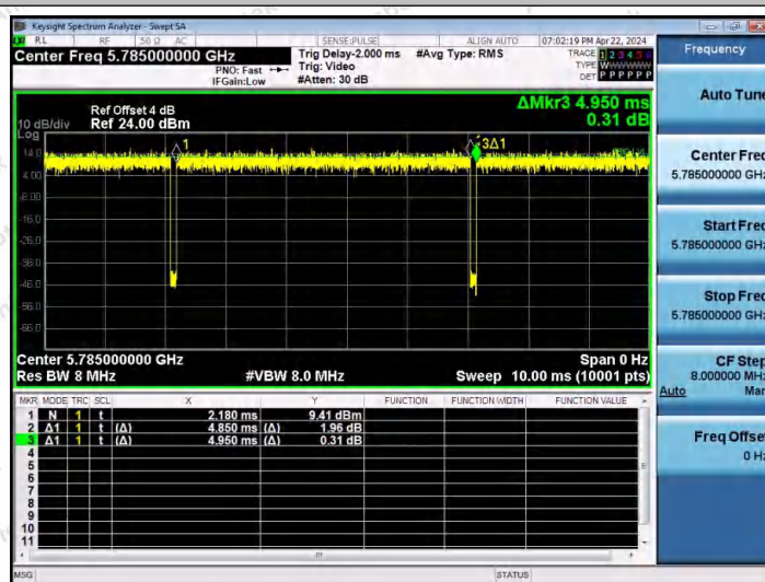
NTNV-11AX20MIMO-Ant1-5785
