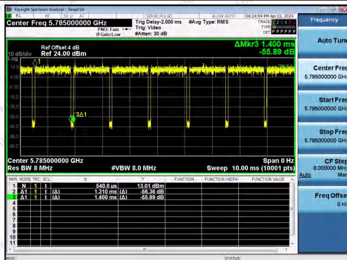
NTNV-11N20MIMO-Ant1-5785
