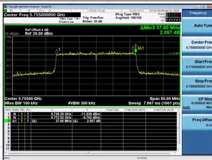
11AX40MIMO-Ant1-5755-PASS
