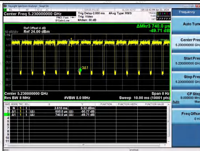
NTNV-11N40MIMO-Ant1-5230
