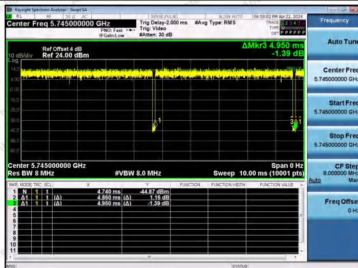
NTNV-11AX20MIMO-Ant1-5745
