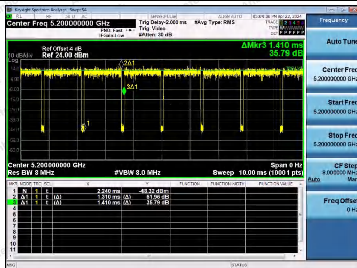
NTNV-11N20MIMO-Ant1-5200
