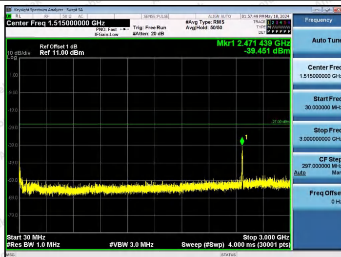
11AX40SISO-Ant1-6405-242Tone-RU62-30~3000-PASS
