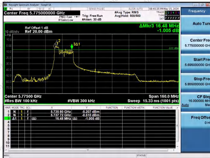
11AX80SISO-Ant1-5775-52Tone-RU37-PASS
