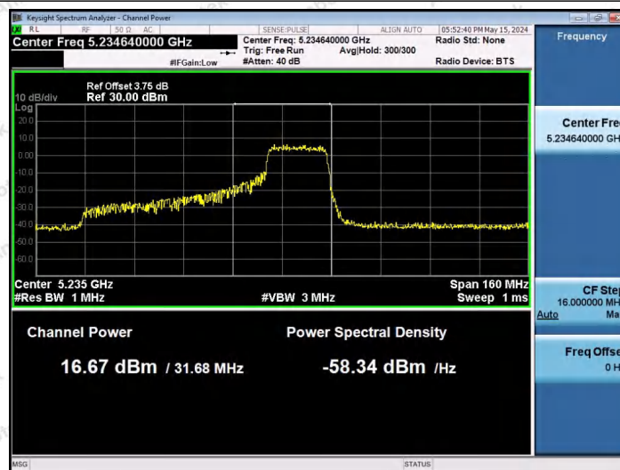
11AX80SISO-Ant1-5210-242Tone-RU64-PASS
