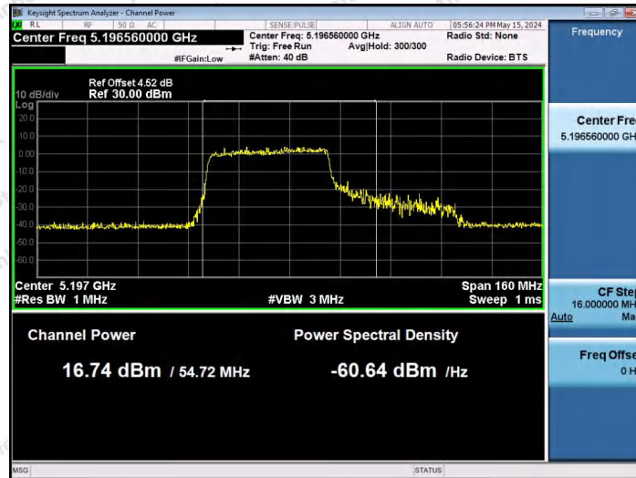
11AX80SISO-Ant1-5210-484Tone-RU65-PASS
