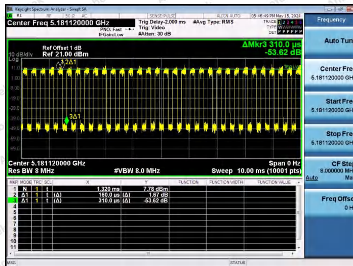
NTNV-11AX80SISO-Ant1-5210-242Tone-RU61
