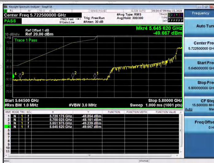
11AX80SISO-Ant1-5775-242Tone-RU64-PASS
