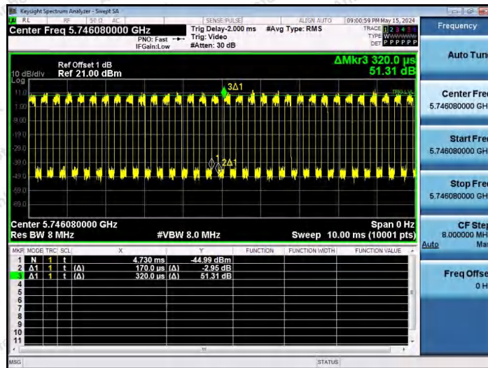
NTNV-11AX80SISO-Ant1-5775-242Tone-RU61
