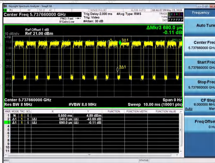
NTNV-11AX80SISO-Ant1-5775-52Tone-RU37
