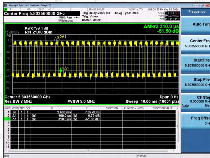
NTNV-11AX80SISO-Ant1-5775-242Tone-RU64
