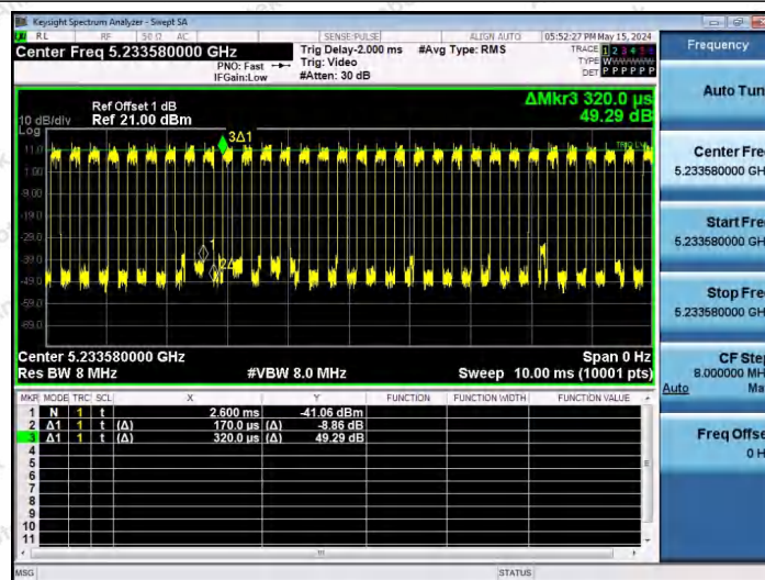
NTNV-11AX80SISO-Ant1-5210-242Tone-RU64
