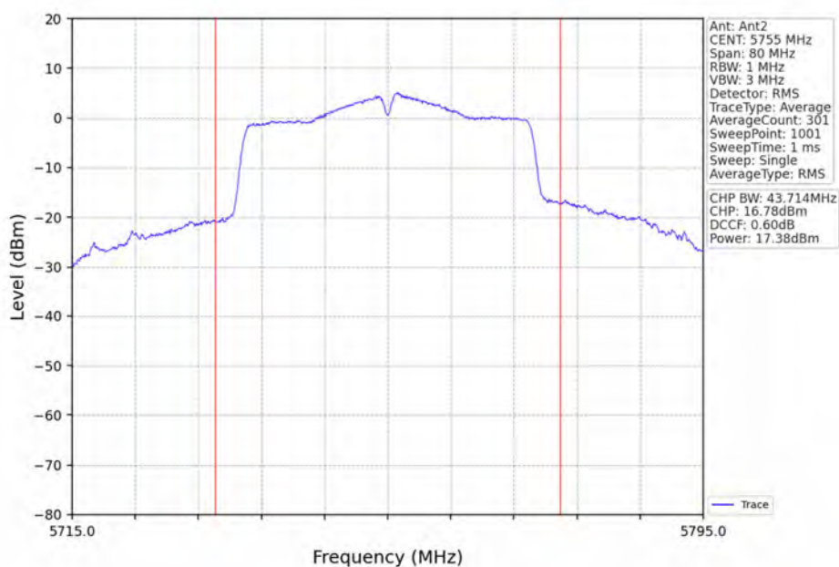
802.11n(HT40)_LCH_5755MHz_Ant2_NTNV
