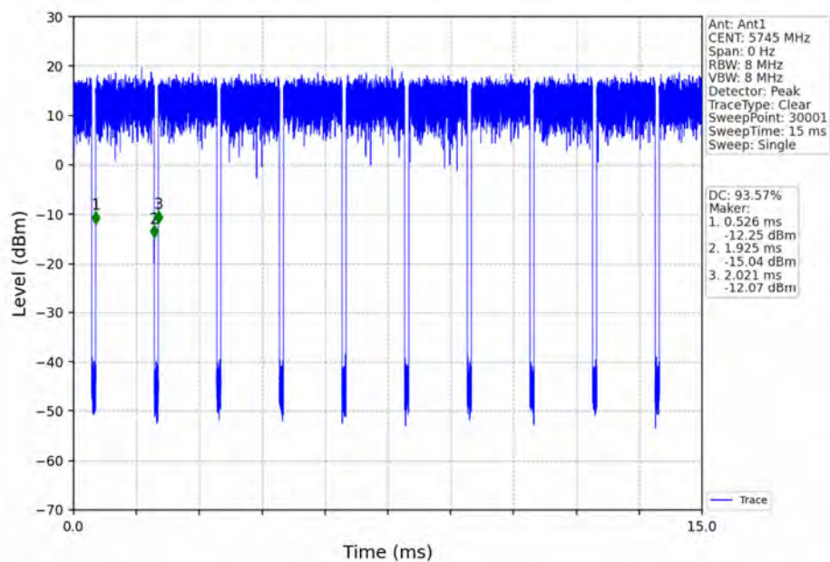
802.11a LCH_5745MHz_Ant1_NTNV
