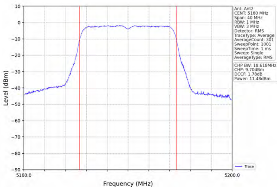
802.11n(HT20)_LCH_5180MHz_Ant2_NTNV
