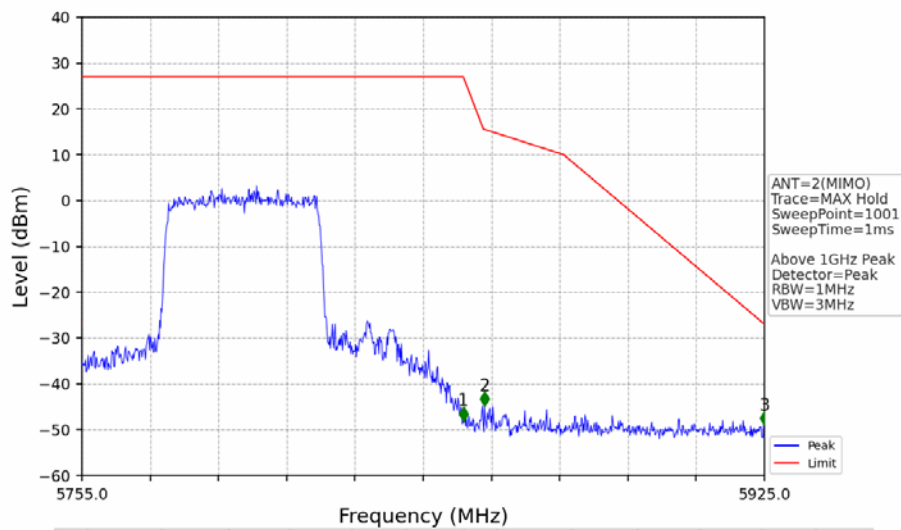
802.11ax(HEW40)_HCH_5795MHz_RU484_Left_Ant2_NTNV
