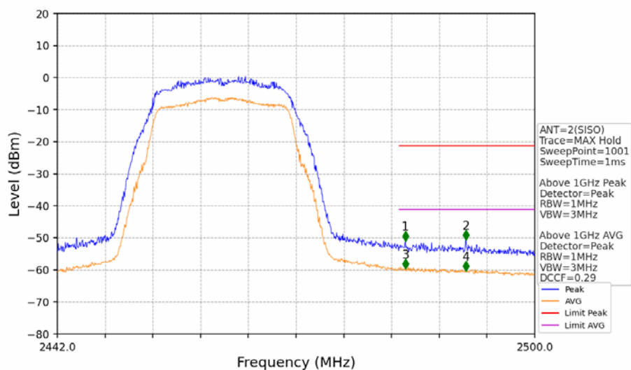
802.11g_HCH_2462MHz_Ant2 (SISO)_NTNV
