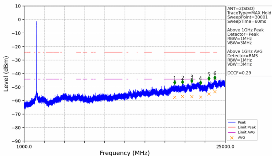
802.11g_HCH_2462MHz_Ant2 (SISO)_NTNV
