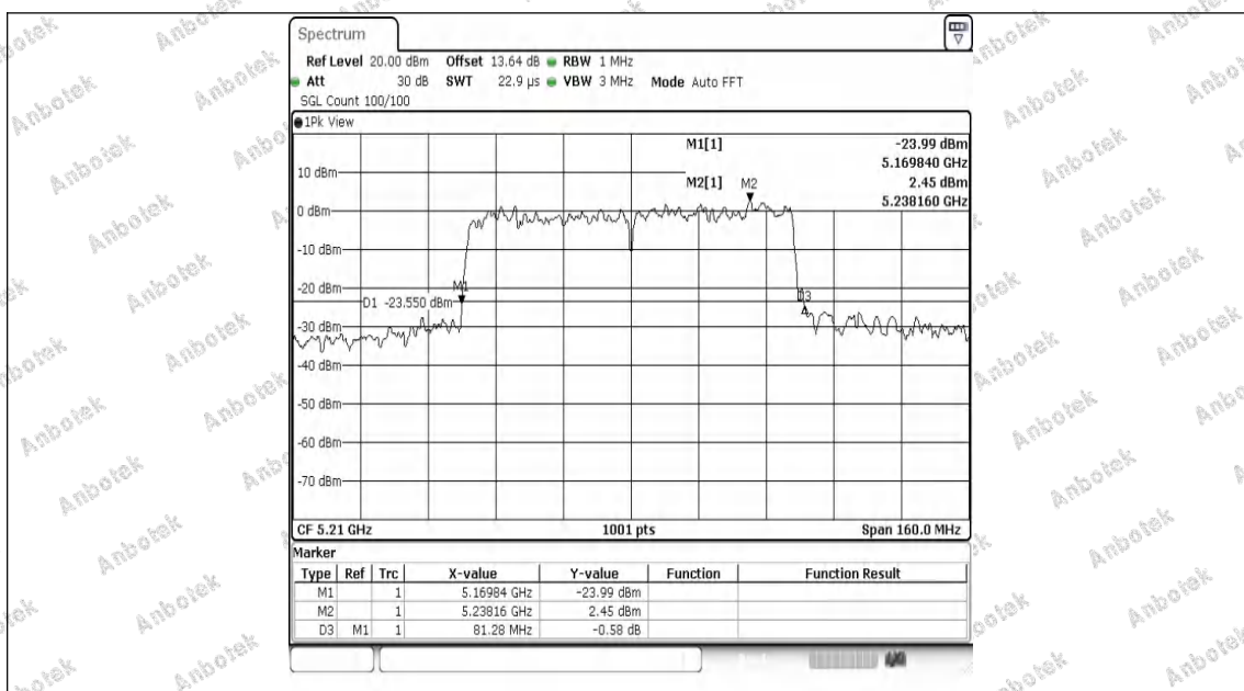
11AC80MIMO-Ant1-5210
