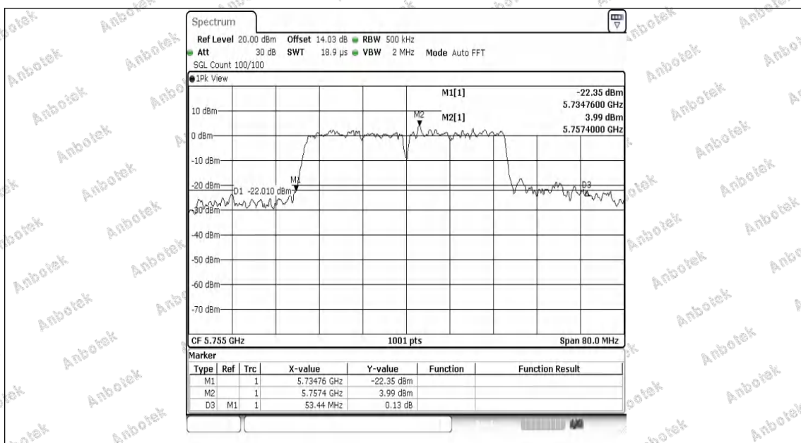
11AC40MIMO-Ant1-5755
