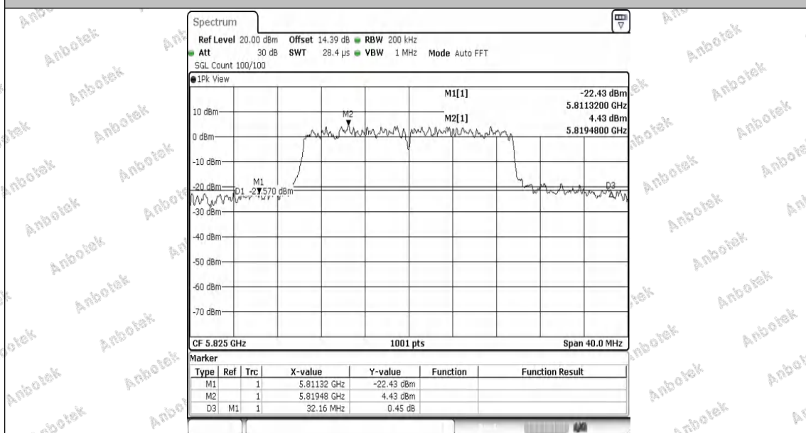
11AX20MIMO-Ant1-5825
