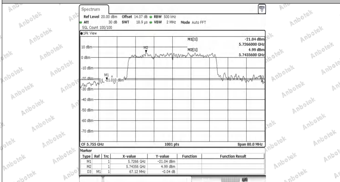
11AX40MIMO-Ant1-5755
