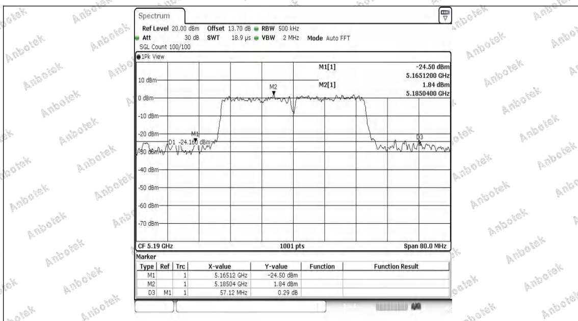
11N40MIMO-Ant1-5190
