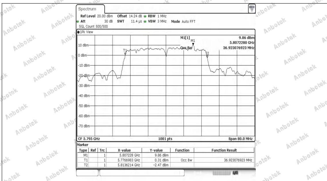
11N40MIMO-Ant1-5795
