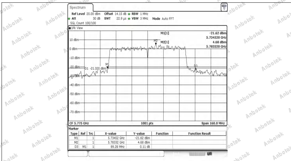
11AC80MIMO-Ant1-5775
