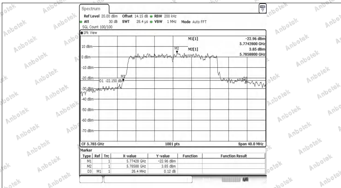
11AX20MIMO-Ant1-5785
