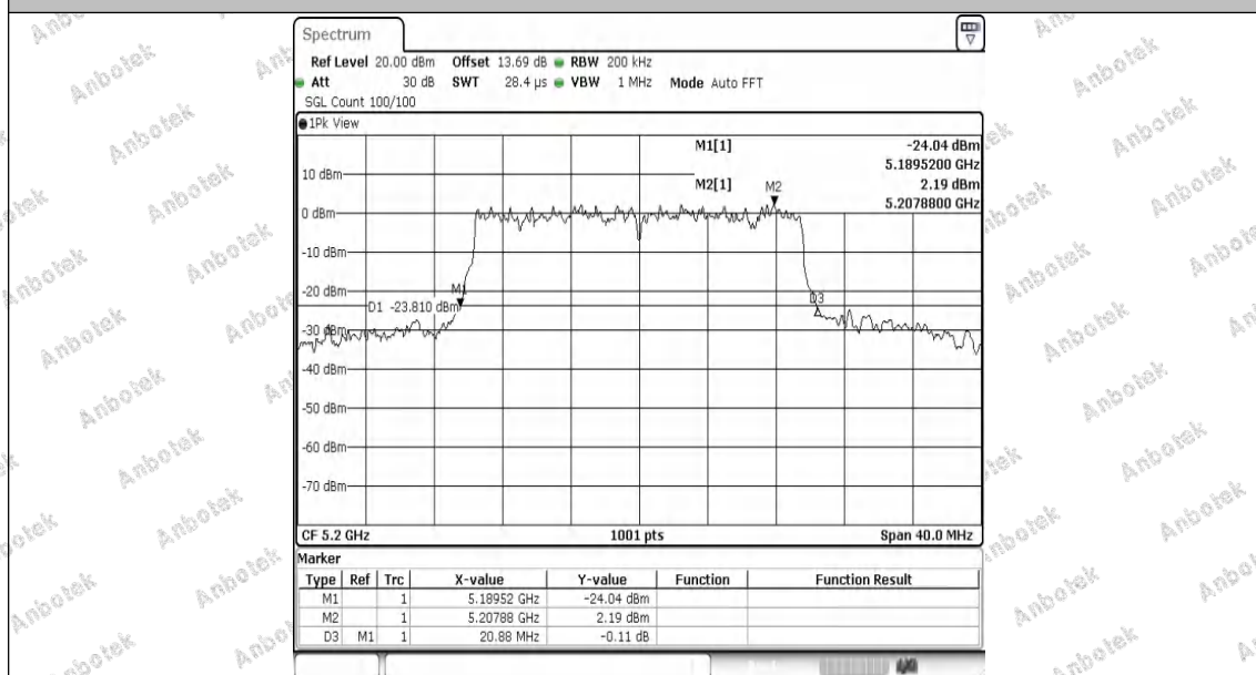
11AX20MIMO-Ant1-5200
