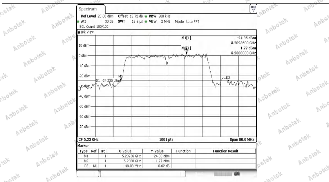
11AC40MIMO-Ant1-5230
