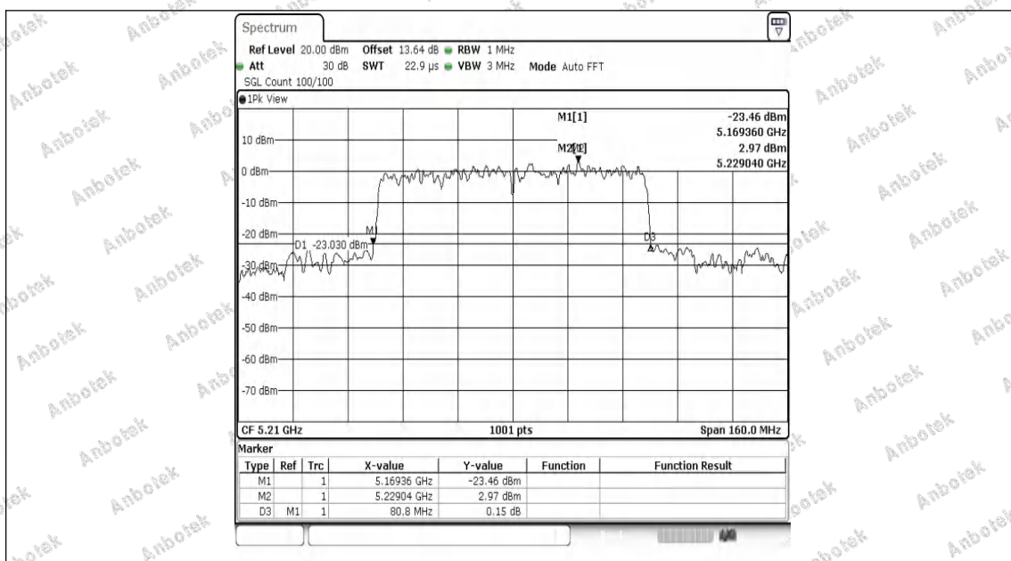
11AX80MIMO-Ant1-5210
