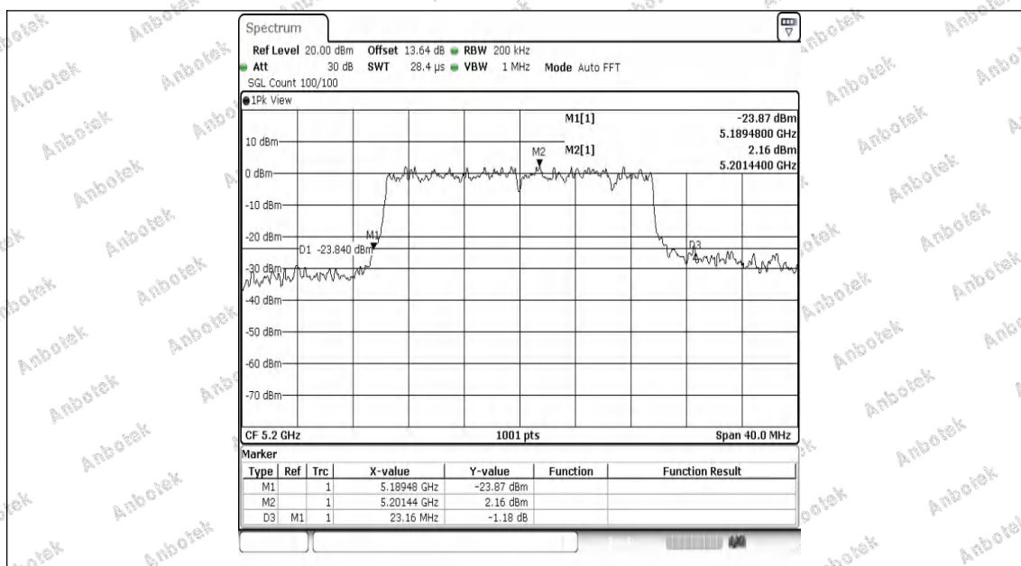
11AX20MIMO-Ant1-5200
