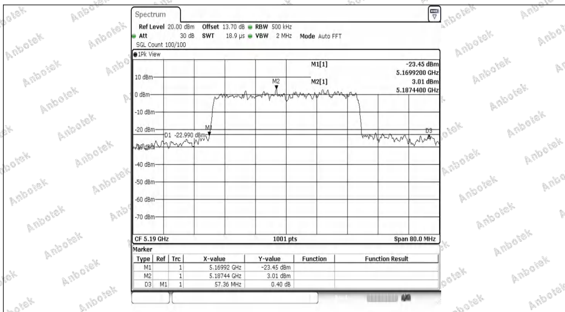
11AX40MIMO-Ant1-5190
