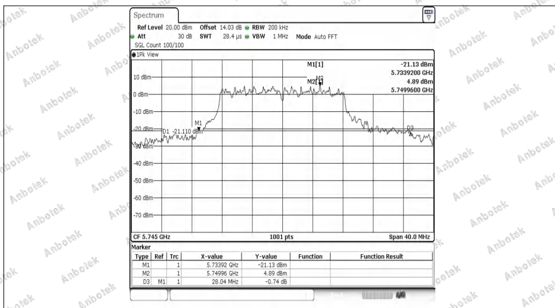
11A-Ant1-5745
