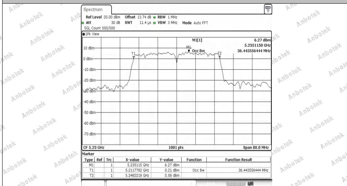
11N40MIMO-Ant1-5230
