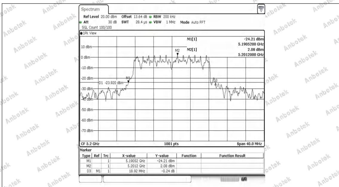
11AC20MIMO-Ant1-5200
