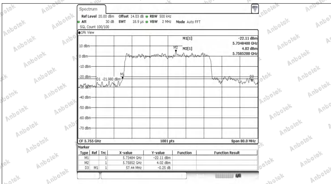
11AX40MIMO-Ant1-5755
