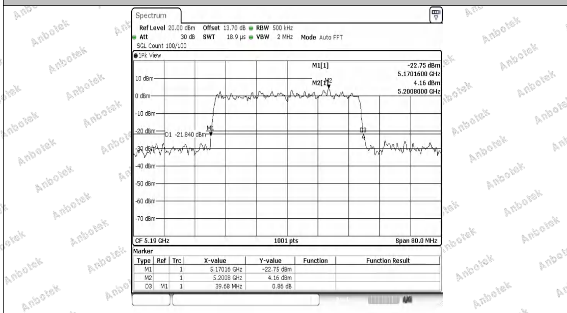
11AX40MIMO-Ant2-5190
