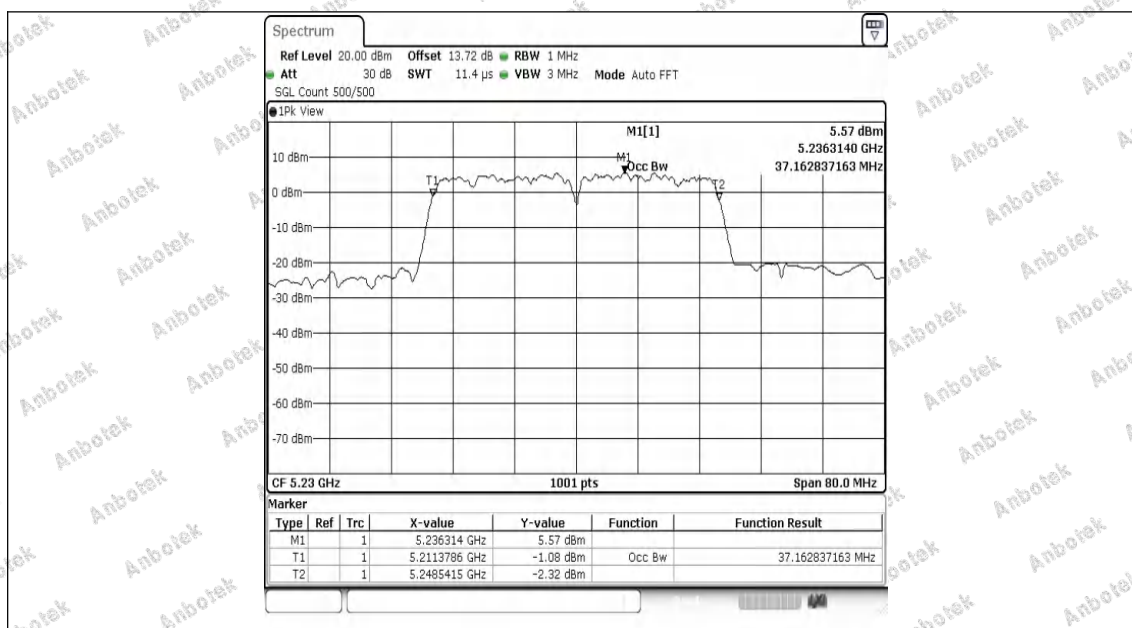
11AC40MIMO-Ant1-5230
