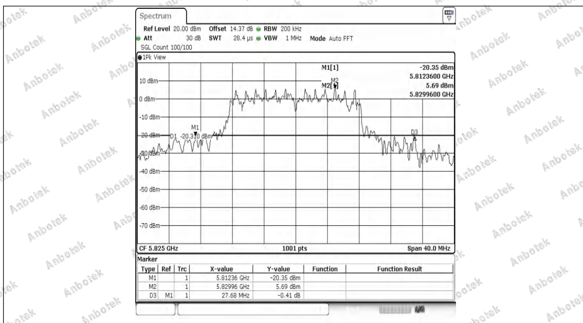
11N20MIMO-Ant1-5825
