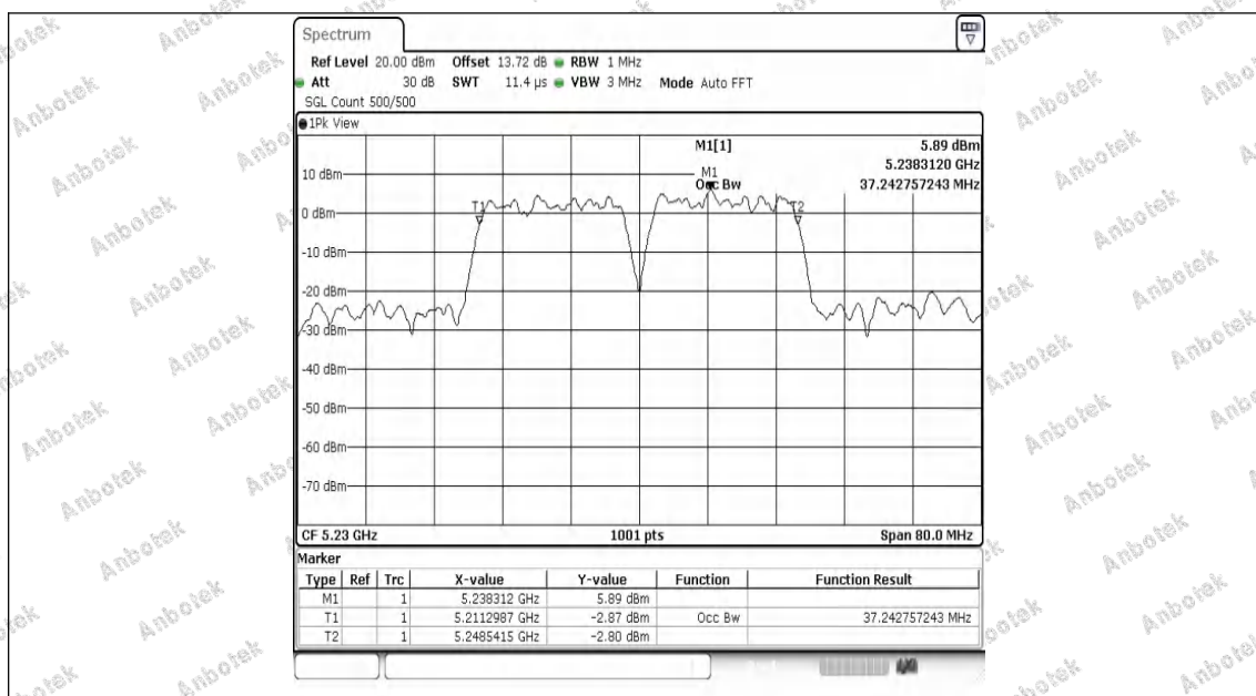
11N40MIMO-Ant1-5230
