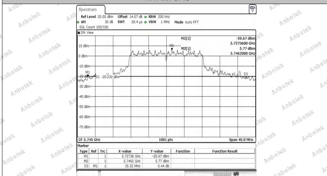
11A-Ant1-5745
