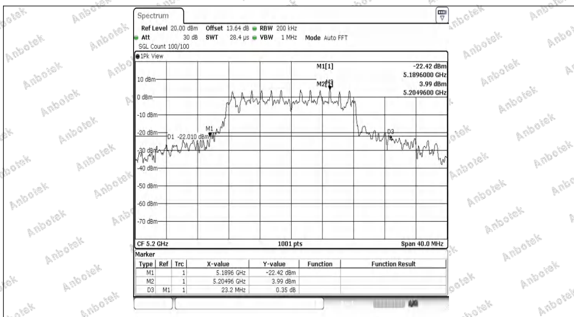
11N20MIMO-Ant1-5200
