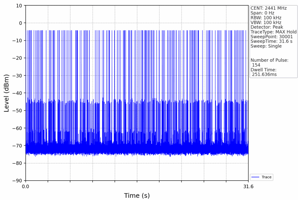
8DPSK_3DH3_HOPP_Ant1_NTNV
