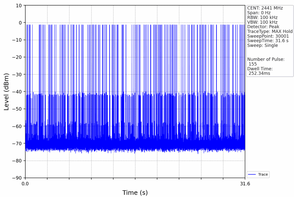
GFSK DH3_HOPP_Ant1_NTNV
