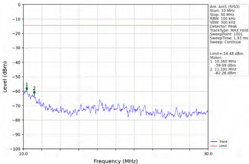
802.11b_HCH_2462MHz_Ant1 (SISO)_NTNV
