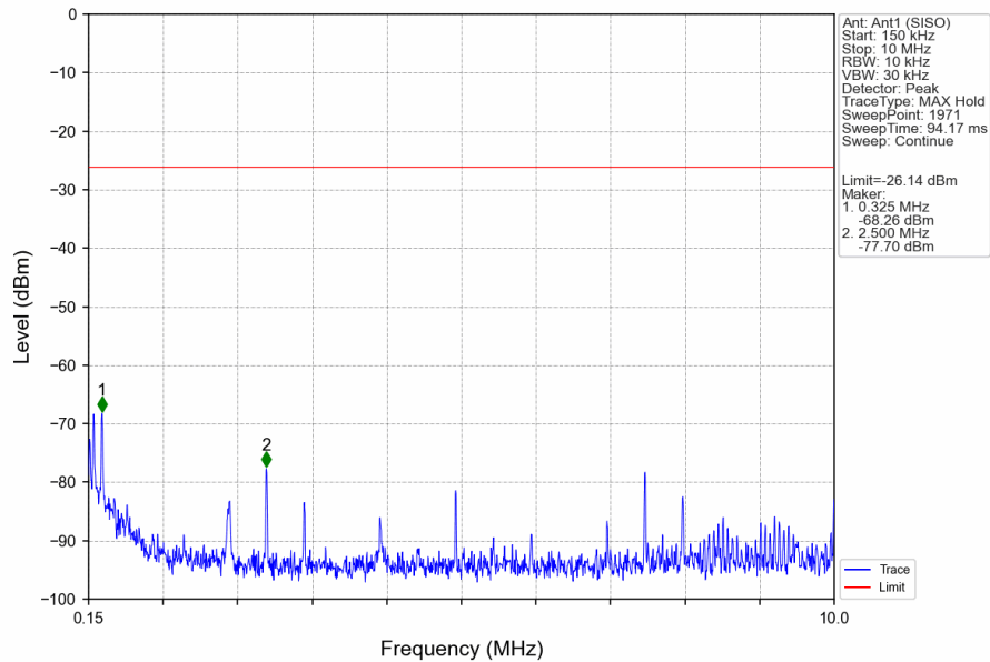
802.11b_LCH_2412MHz_Ant1 (SISO)_NTNV
