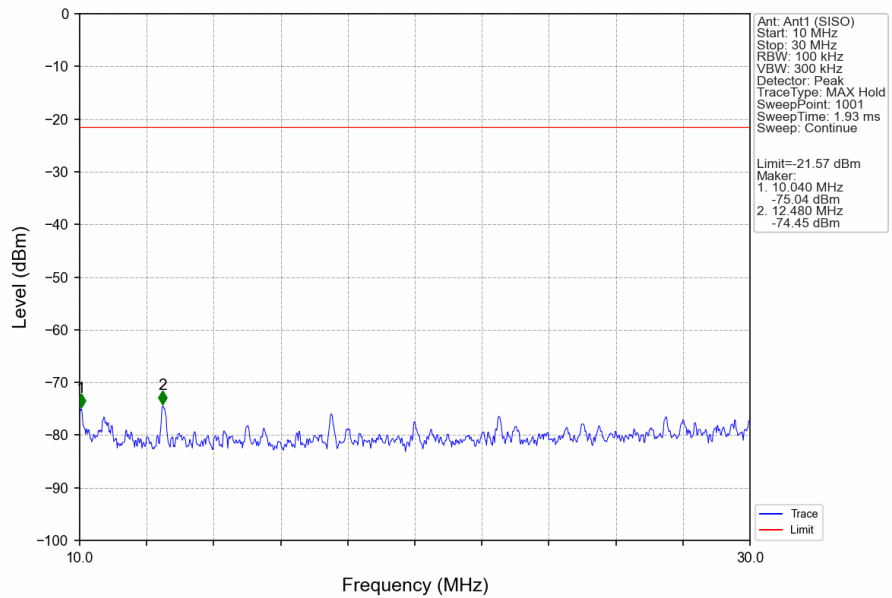
802.11g_LCH_2412MHz_Ant1 (SISO)_NTNV
