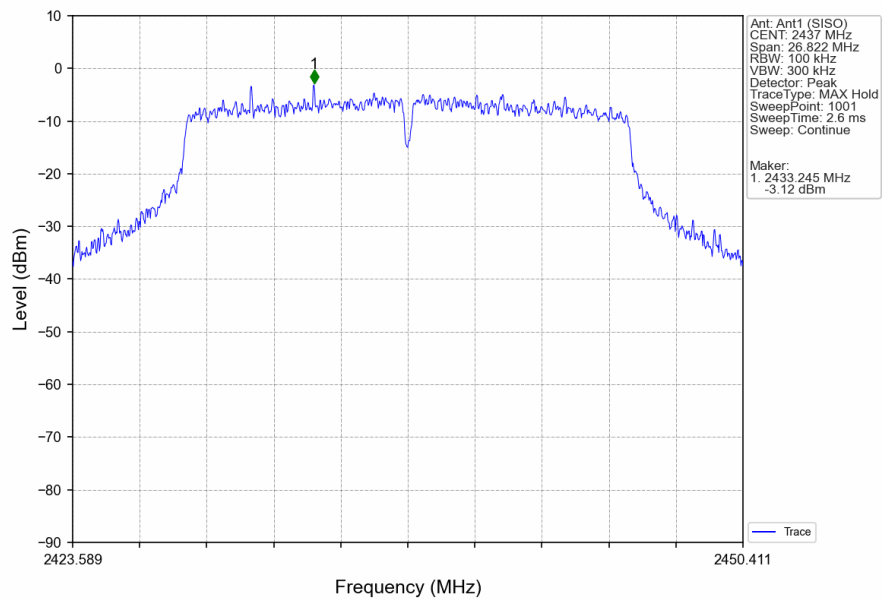
802.11n(HT20)_MCH_2437MHz_Ant1 (SISO)_NTNV
