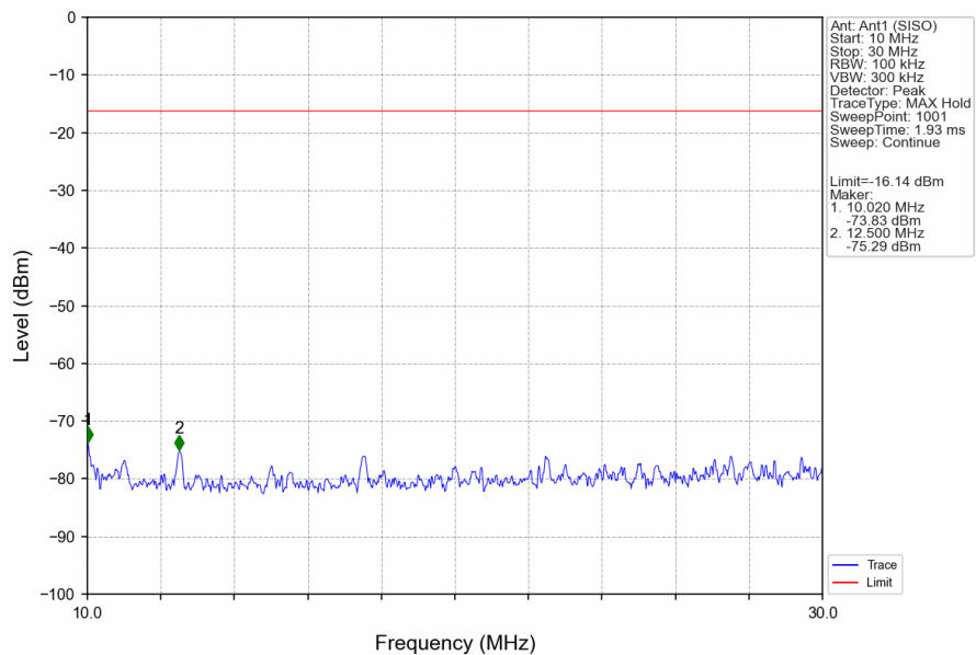
802.11b_LCH_2412MHz_Ant1 (SISO)_NTNV
