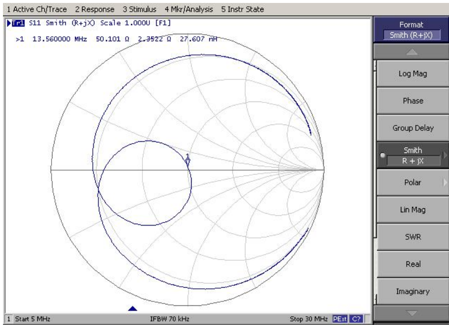
史密斯图
