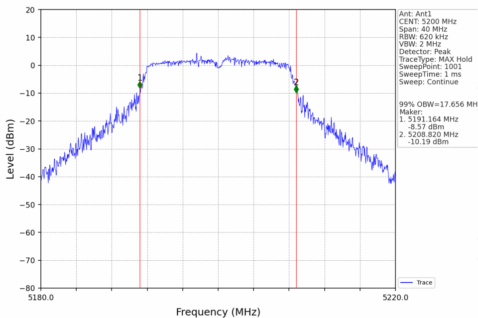
802.11a_MCH_5200MHz_Ant1_NTNV
