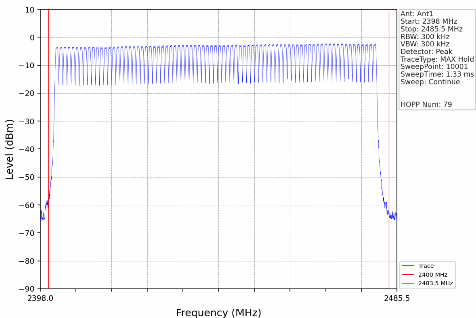
Pi/4DQPSK_2DH5_HOPP_Ant1_NTV
