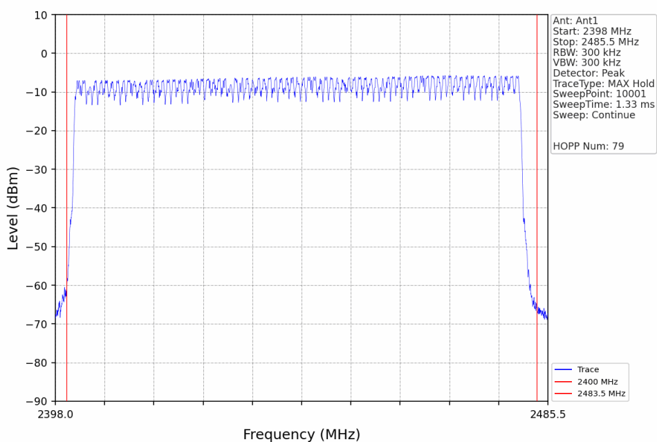
Pi/4DQPSK_2DH5_HOPP_Ant1_NTV
