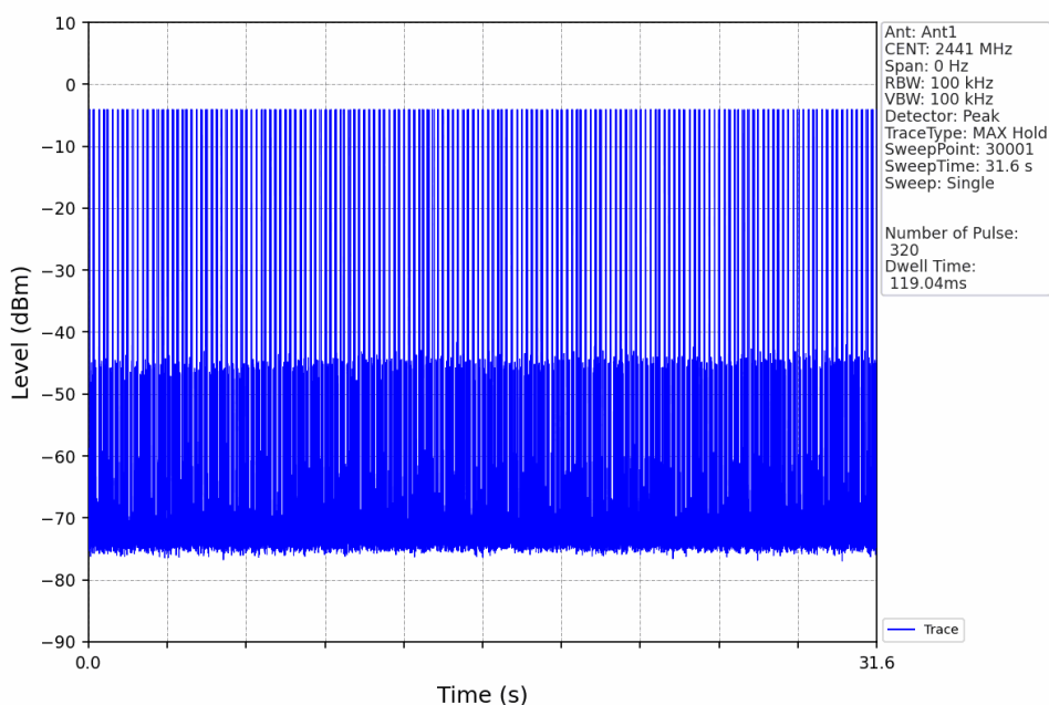
GFSK_DH1_HOPP_Ant1_NTNV
