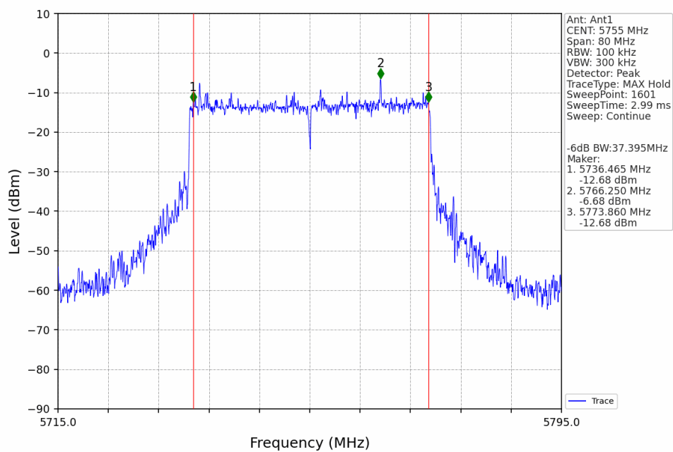
802.11ax(HEW40) LCH 5755MHz SU / Ant1 NTNV
