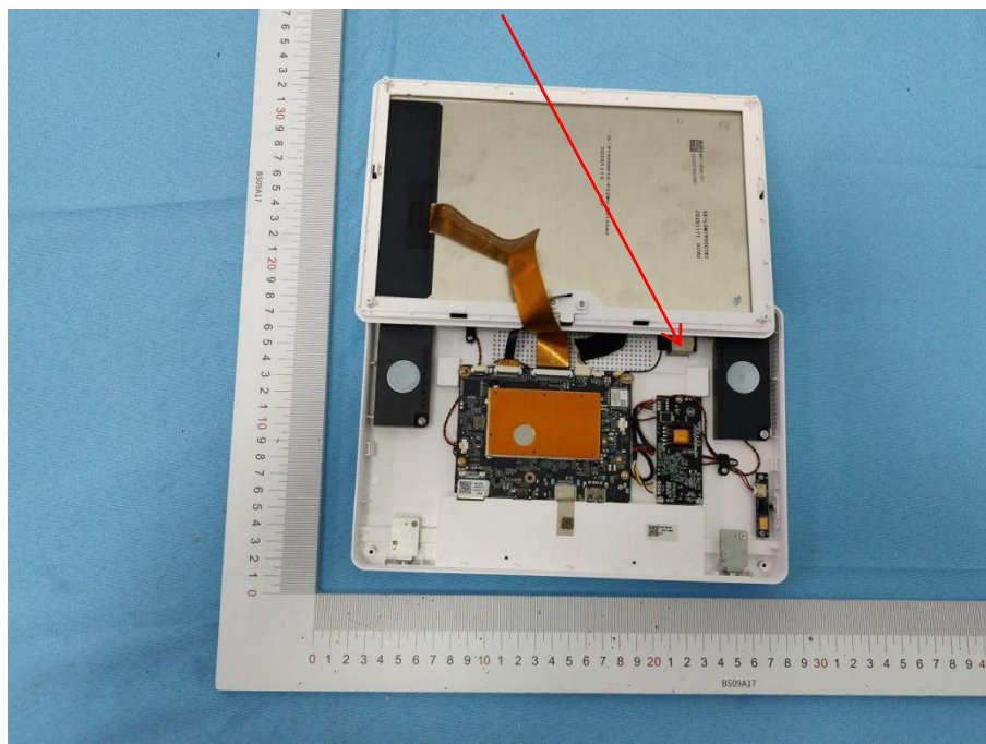
BT&BLE&WiFi-ANT
