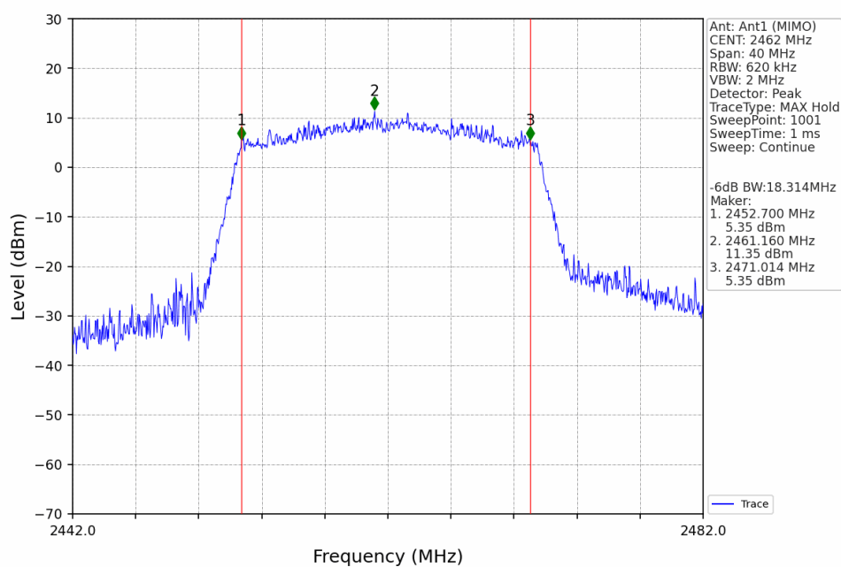
802.11ax(HEW20) HCH 2462MHz SU / Ant1 (MIMO) NTN
