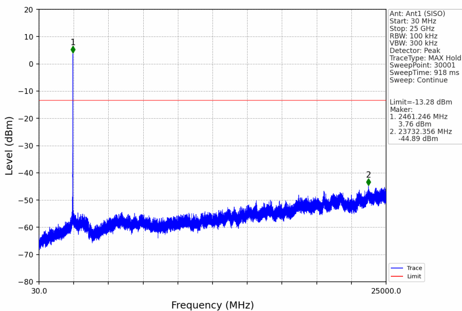
802.11b HCH 2462MHz Ant1 (SISO) NTV
