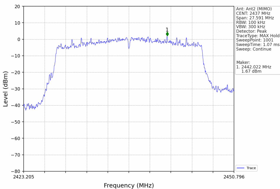
802.11ax(HEW20) MCH 2437MHz SU / Ant2 (MIMO) NTN
