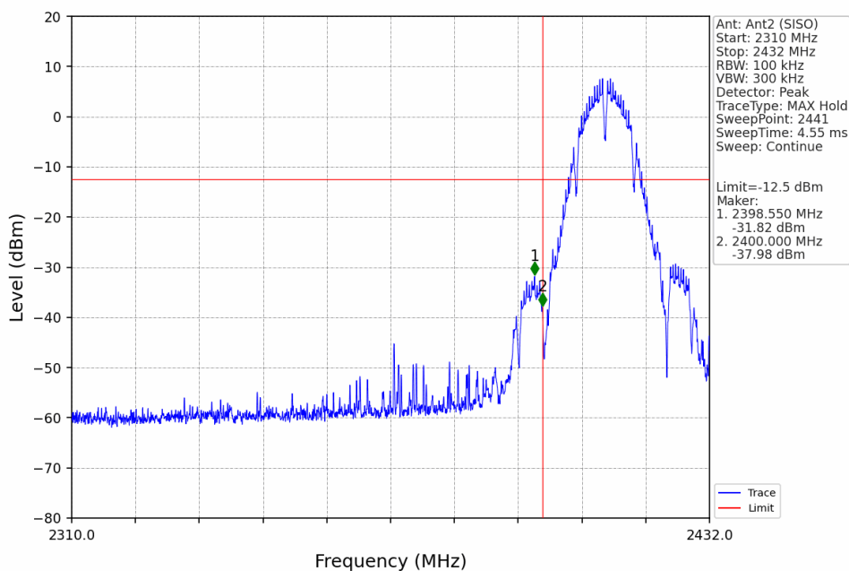
802.11b LCH 2412MHz Ant2 (SISO) NTV
