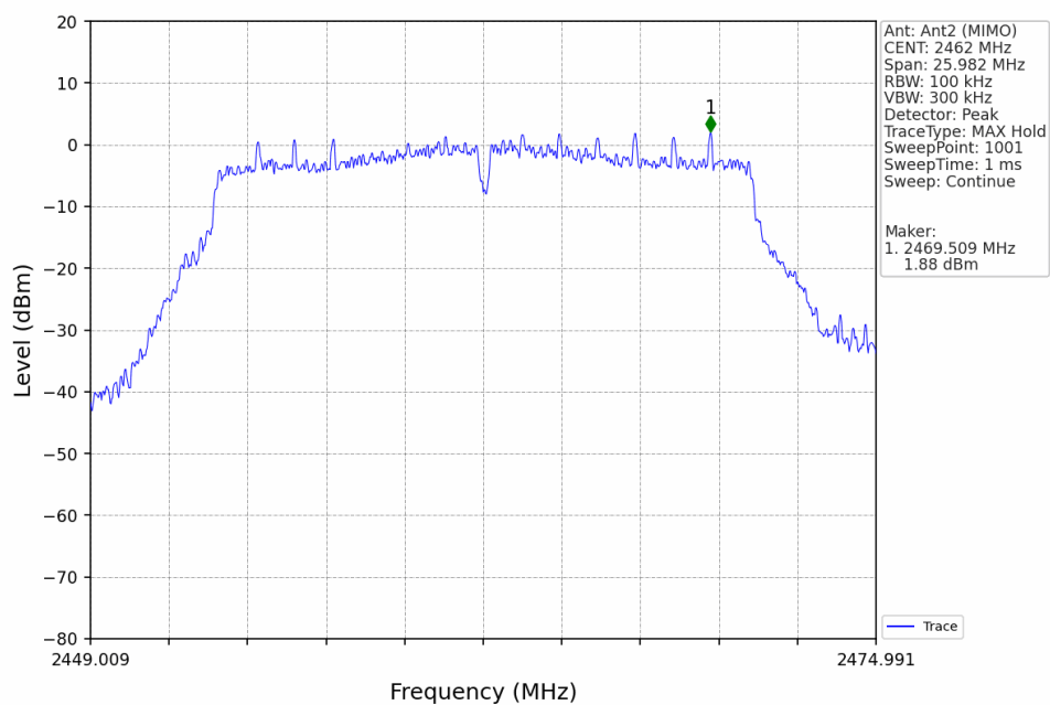
802.11n(HT20) HCH 2462MHz Ant2 (MIMO) NTV
