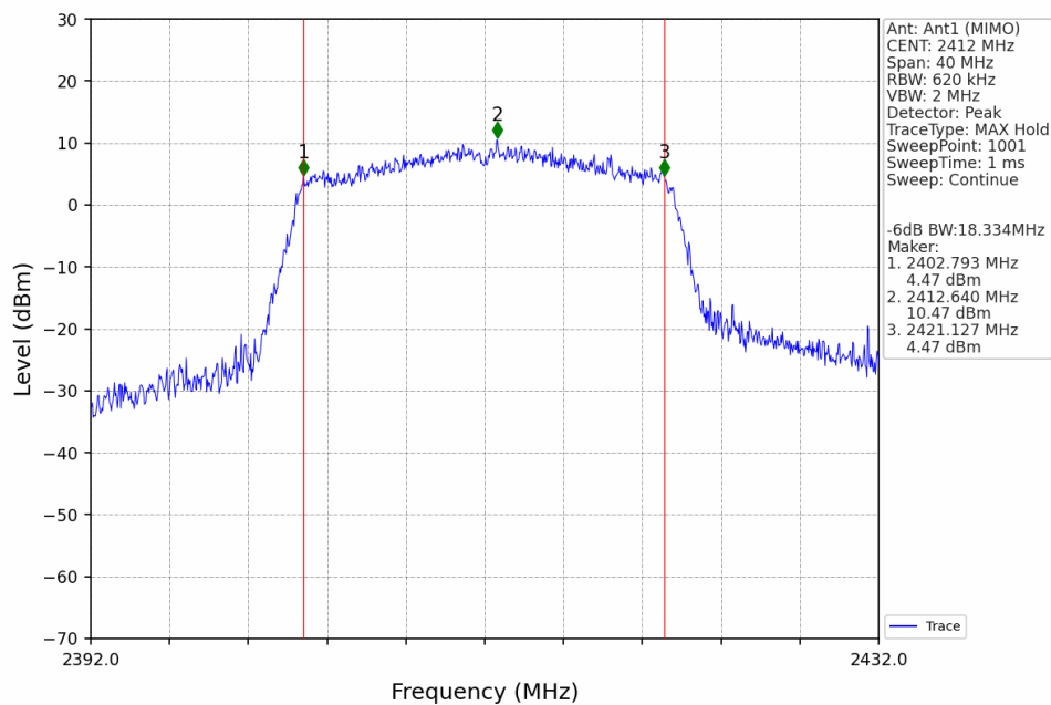
802.11ax(HEW20) LCH 2412MHz SU / Ant1 (MIMO) NTN
