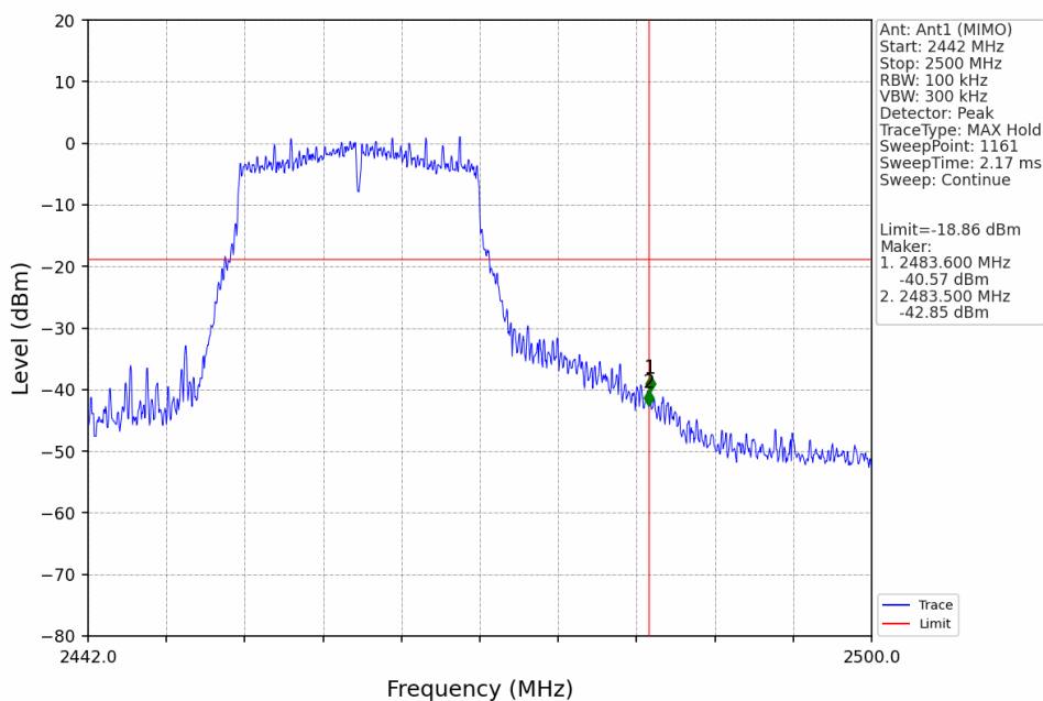
802.11n(HT20) HCH 2462MHz Ant1 (MIMO) NTVN
