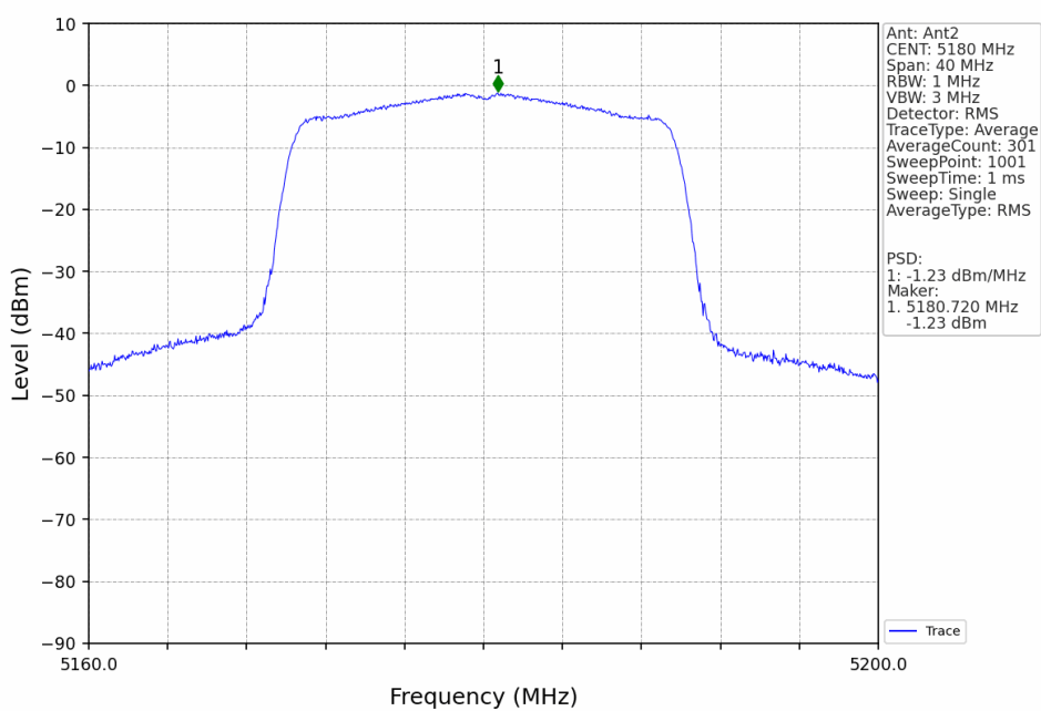
802.11ax(HEW20) LCH 5180MHz SU / Ant2 NTV
