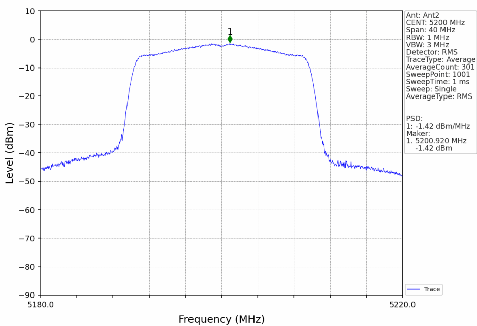
802.11ax(HEW20) MCH 5200MHz SU / Ant2 NTN
