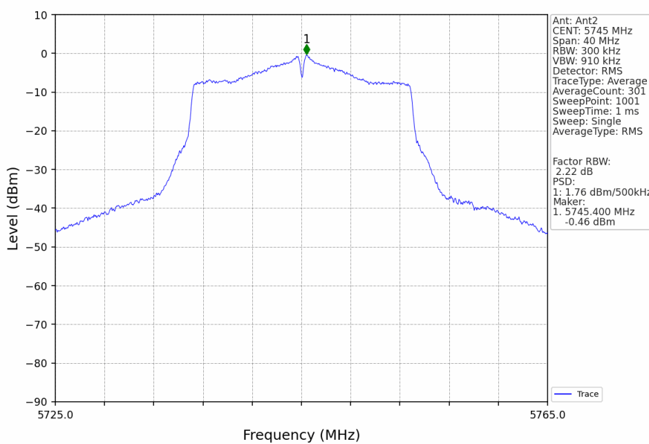
802.11n(HT20) LCH 5745MHz_Ant2_NTNV
