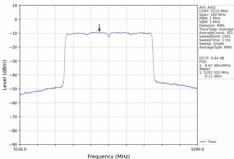
802.11ax(HEW80) MCH 5210MHz SU / Ant2 NTN
