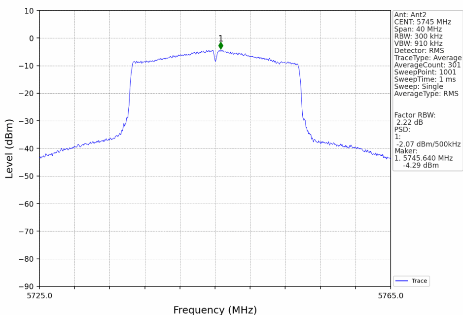
802.11ax(HEW20) LCH 5745MHz SU / Ant2 NTNV
