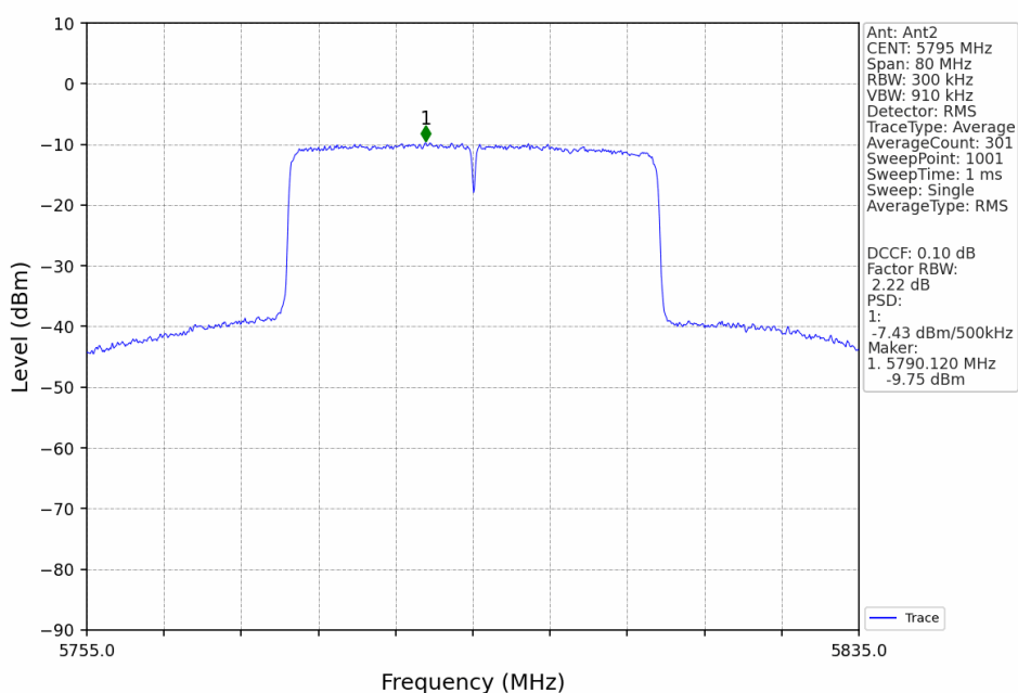
802.11ax(HEW40) HCH 5795MHz SU / Ant2 NTN
