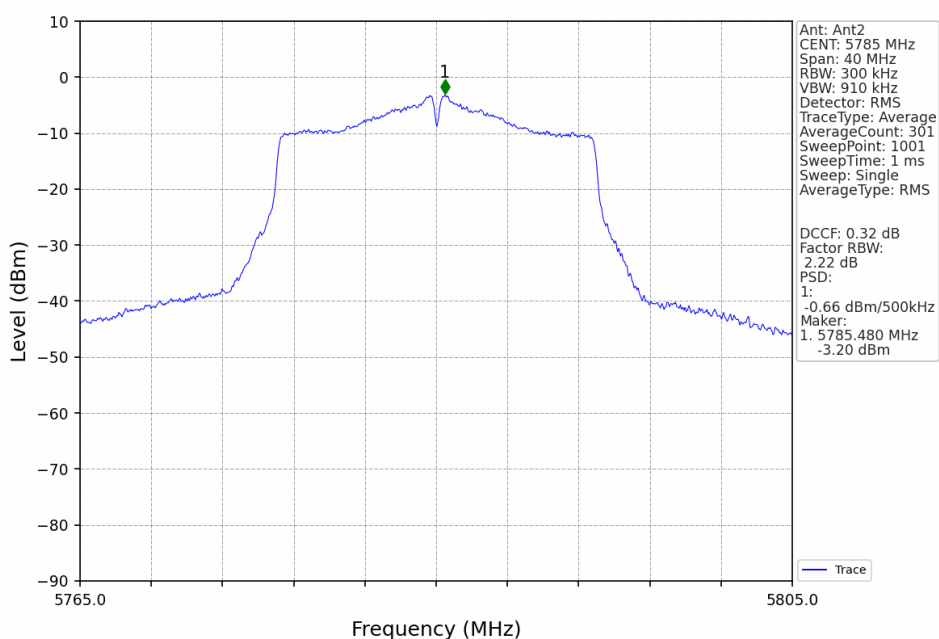
802.11ac(VHT20) MCH 5785MHz_Ant2_NTNV
