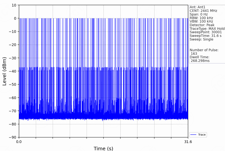
GFSK_DH3_HOPP_Ant1_NTNV
